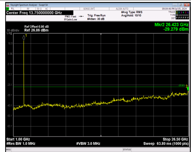
Band41-20MHz-QPSK-40640-1RB#0-Range2:1000~26 500MHz
