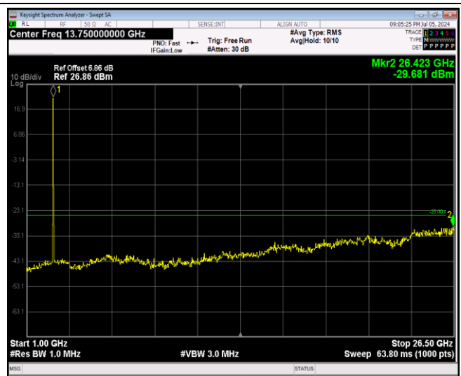
Band41-20MHz-QPSK-41140-1RB#0-Range2:1000~26500MHz
