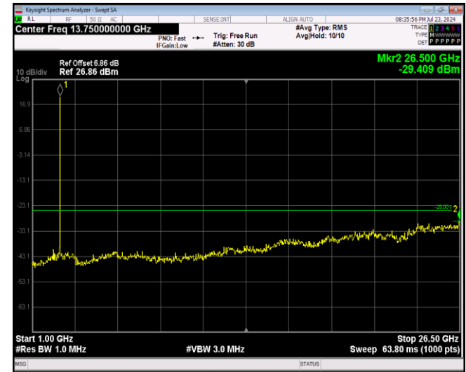
Band41-20MHz-QPSK-40140-1RB#0-Range2:1000~26 500MHz
