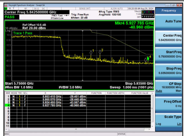
11AX80SISO-Ant2-5775-PASS
