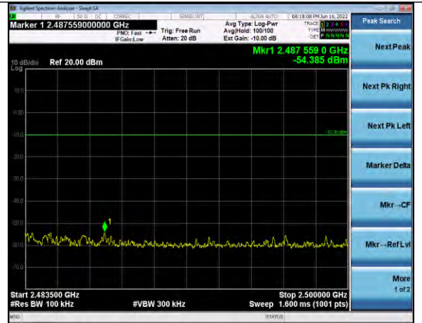
DH5 Hopping
