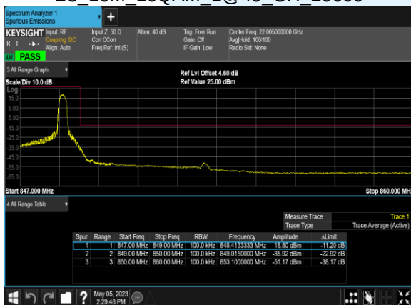
B5 10M 16QAM 1@49 CH 20600
