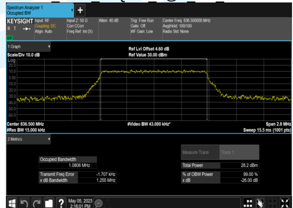
B5 1.4M 16QAM 6@0 CH 20525
