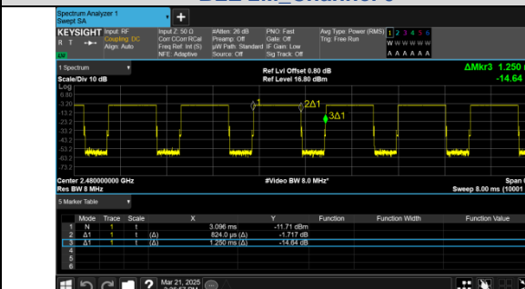
BLE 2M_Channel 39
