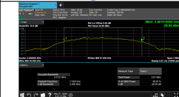
BLE 2M_Channel 39
