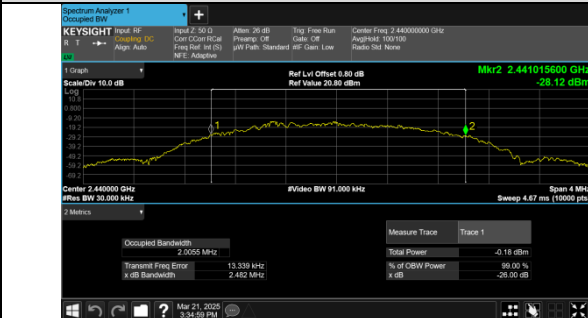
BLE 2M_Channel 19
