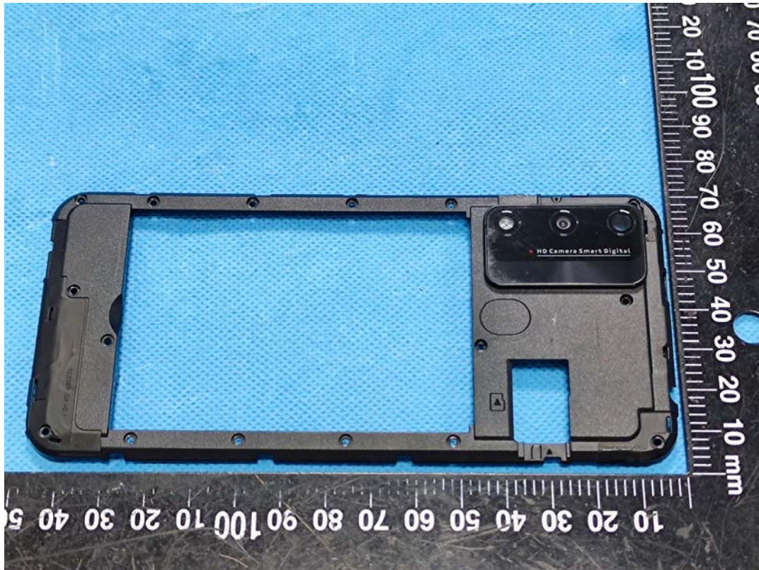
BT/WiFi/GPS Antenna
