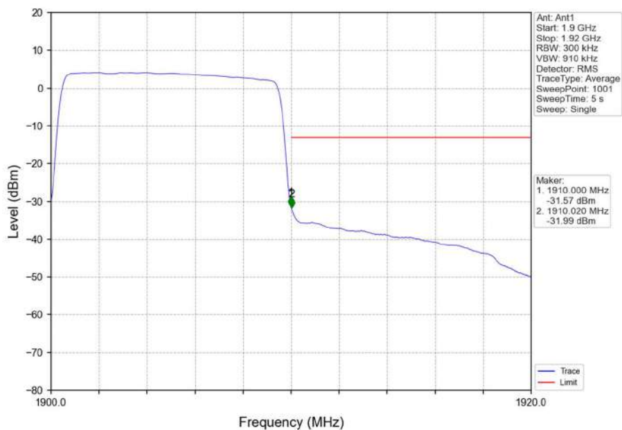
Band2_10MHz_16QAM_HCH_1905MHz_RB_50_0_NTNV
