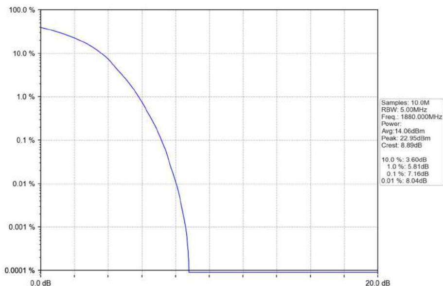
Band2_20MHz_QPSK_MCH_1880MHz_RB_100_0_NTNV
