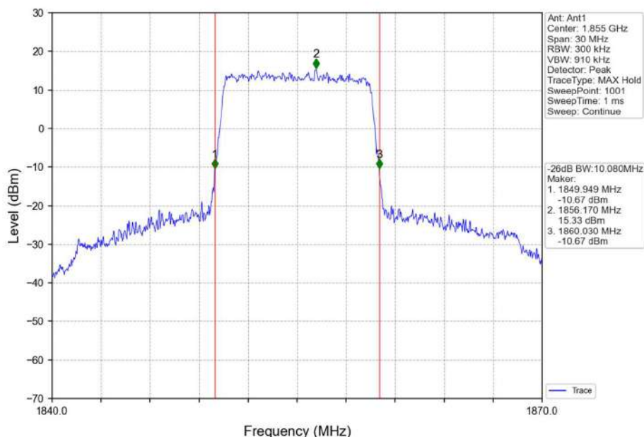
Band2_10MHz_QPSK_LCH_1855MHz_RB_50_0_NTNV
