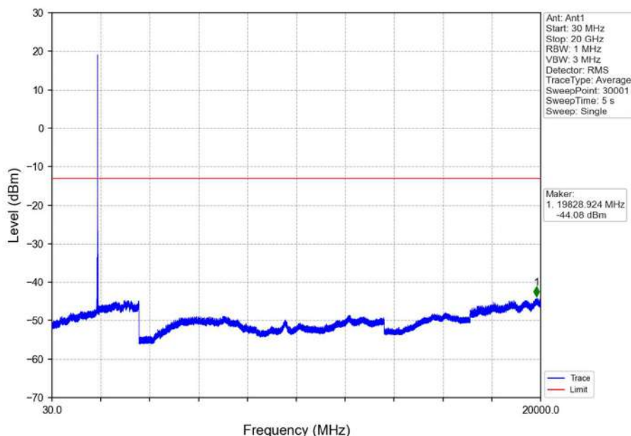
Band2_15MHz_QPSK_HCH_1902.5MHz_RB_1_0_NTNV
