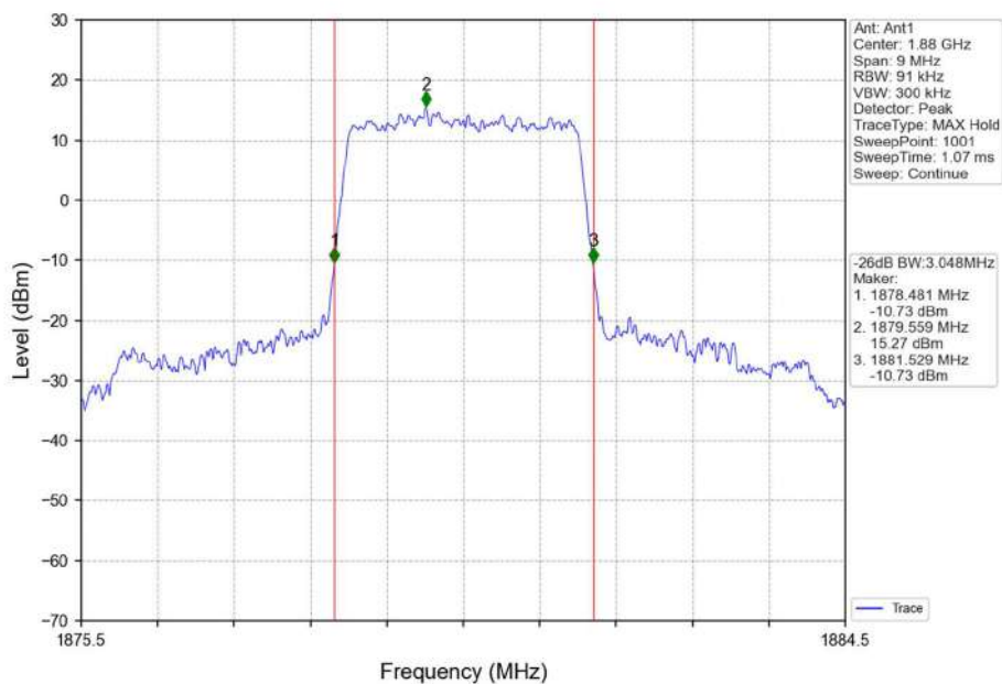
Band2_3MHz_QPSK_MCH_1880MHz_RB_15_0_NTNV
