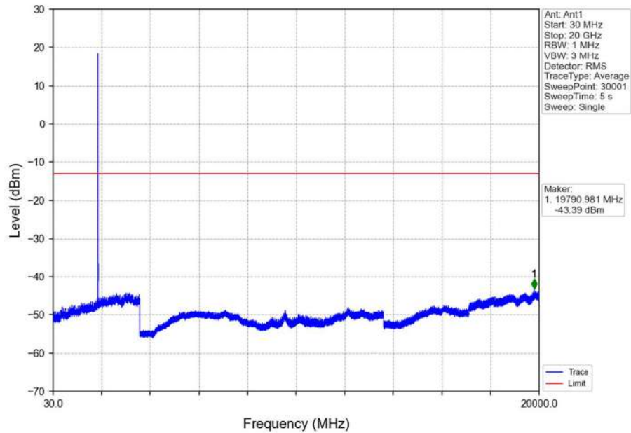
Band2_3MHz_16QAM_MCH_1880MHz_RB_1_0_NTNV
