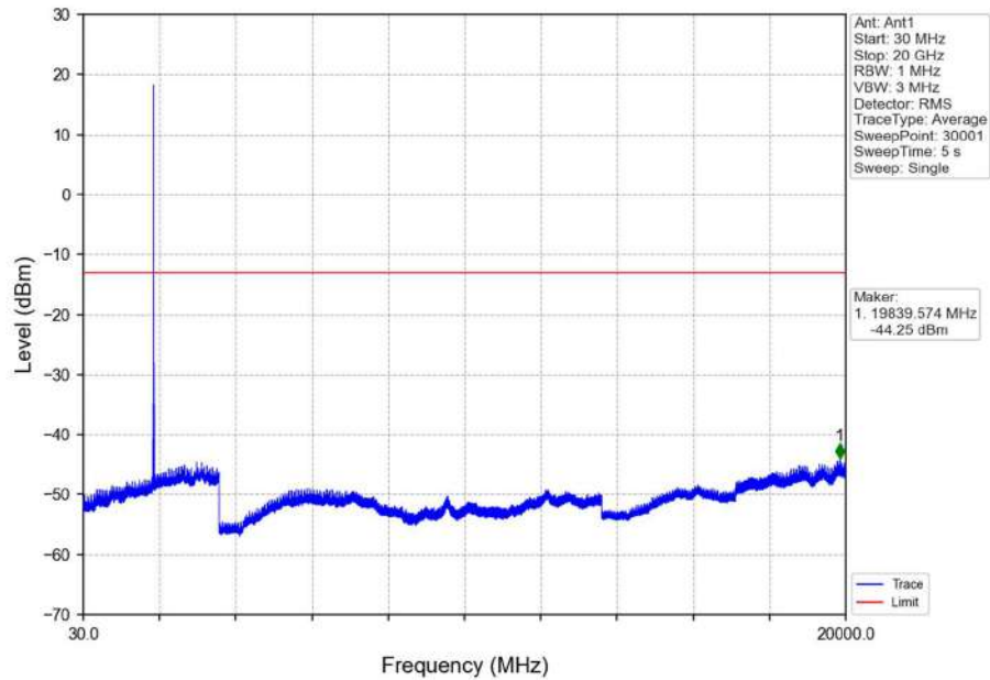
Band2_10MHz_16QAM_MCH_1880MHz_RB_1_0_NTNV
