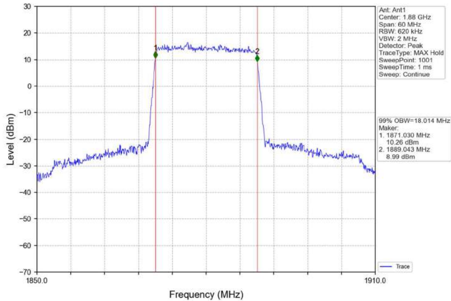
Band2_20MHz_QPSK_MCH_1880MHz_RB_100_0_NTNV
