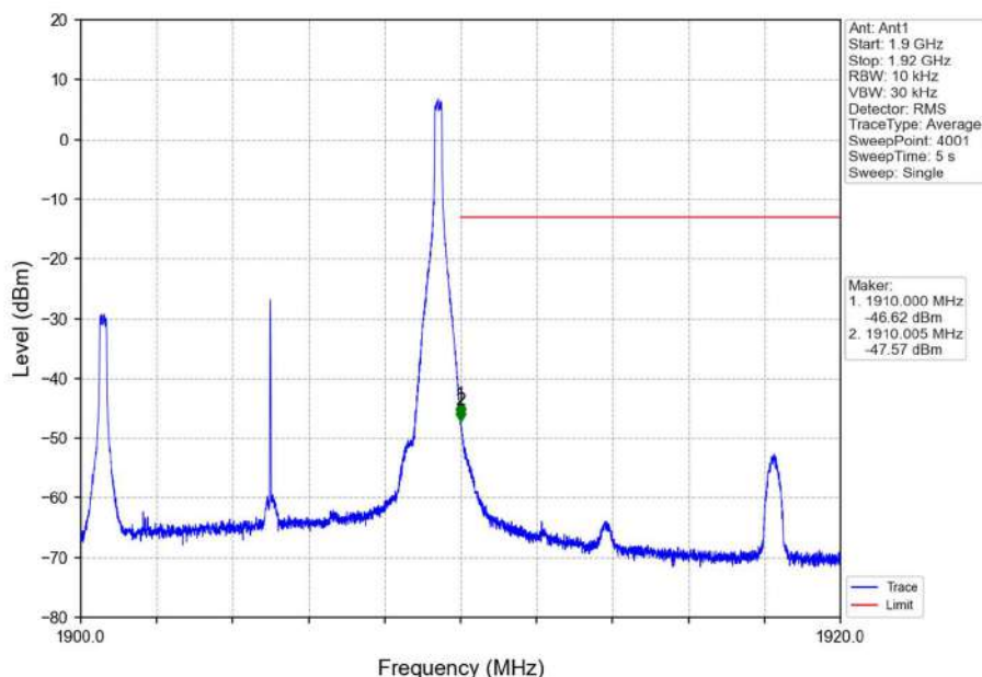
Band2_10MHz_16QAM_HCH_1905MHz_RB_1_49_NTNV
