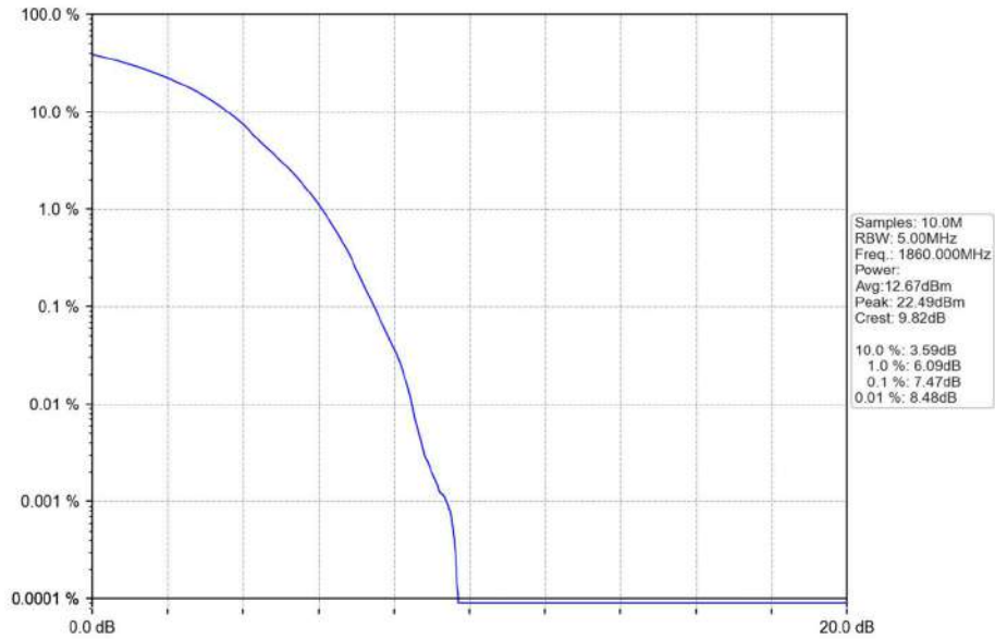
Band2_20MHz_16QAM_LCH_1860MHz_RB_100_0_NTNV
