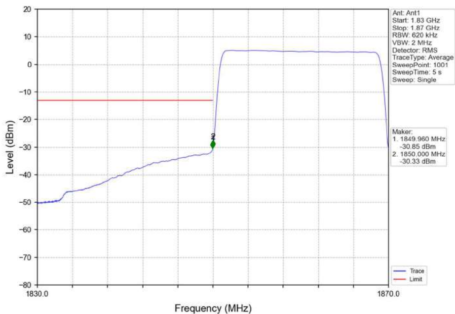
Band2_20MHz_QPSK_LCH_1860MHz_RB_100_0_NTNV
