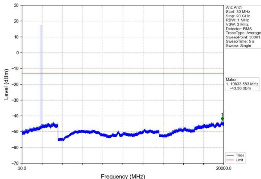
Band2_1.4MHz_QPSK_HCH_1909.3MHz_RB_1_0_NTNV
