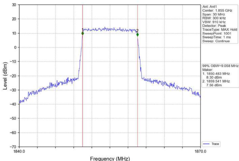
Band2_10MHz_16QAM_LCH_1855MHz_RB_50_0_NTNV
