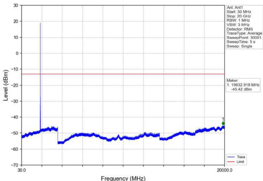
Band2_10MHz_QPSK_MCH_1880MHz_RB_1_0_NTNV
