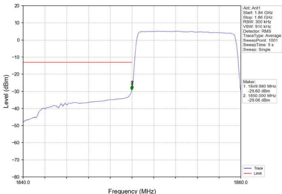
Band2_10MHz_QPSK_LCH_1855MHz_RB_50_0_NTNV
