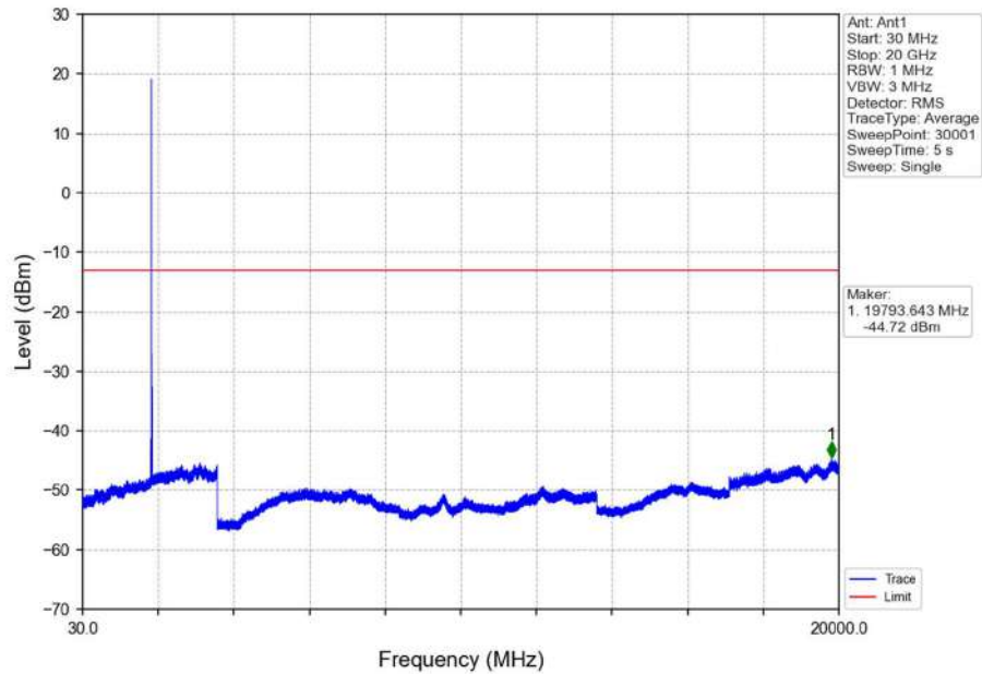
Band2_10MHz_16QAM_LCH_1855MHz_RB_1_0_NTNV
