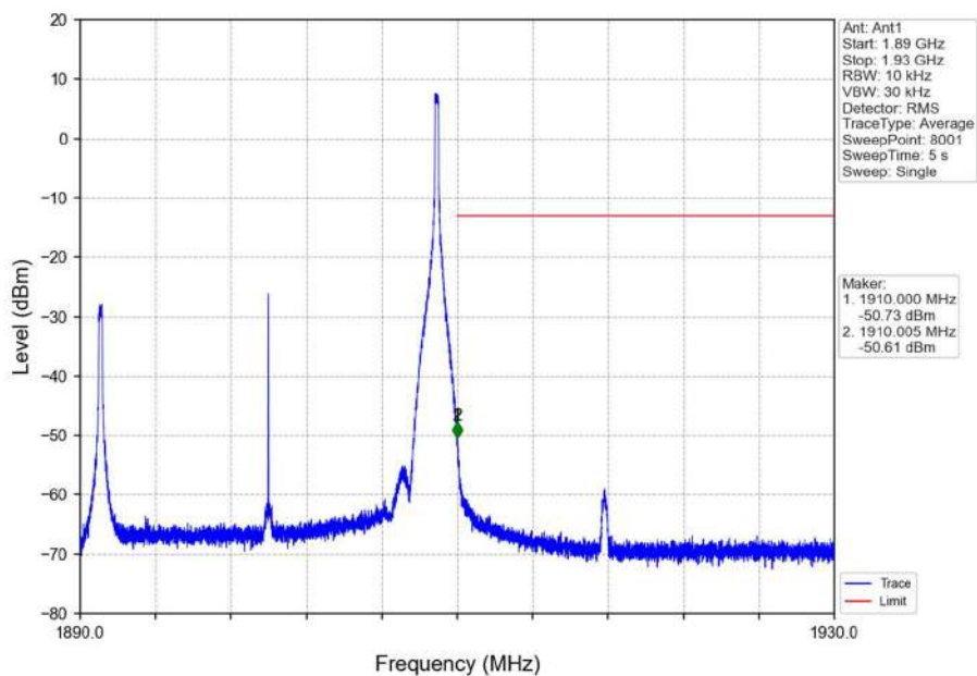
Band2_20MHz_QPSK_HCH_1900MHz_RB_1_99_NTNV
