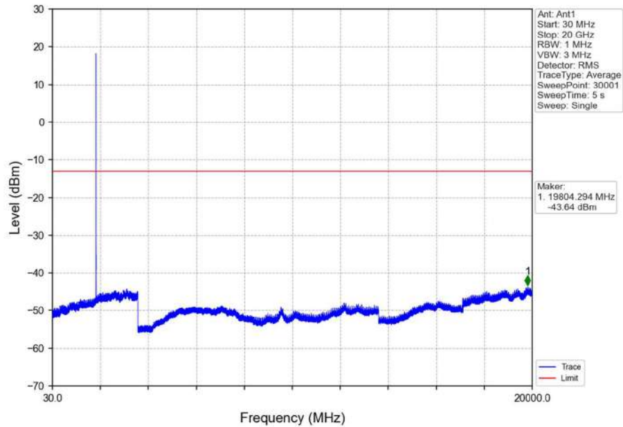
Band2_3MHz_QPSK_LCH_1851.5MHz_RB_1_0_NTNV
