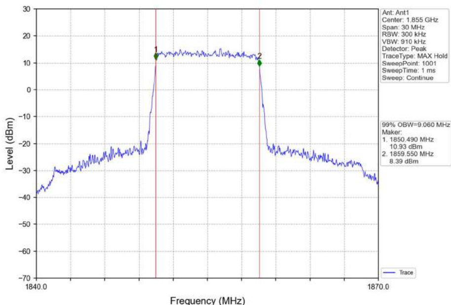
Band2_10MHz_QPSK_LCH_1855MHz_RB_50_0_NTNV
