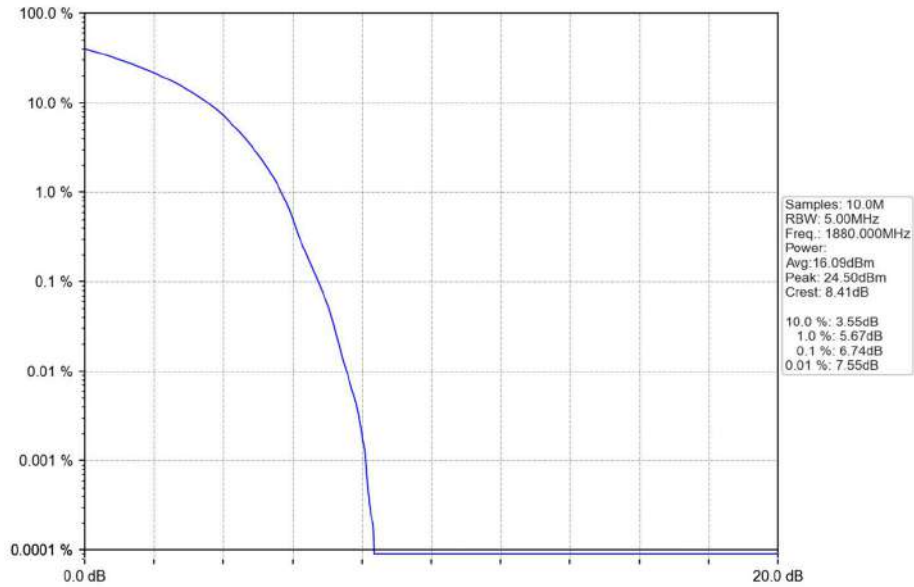
Band2_10MHz_16QAM_MCH_1880MHz_RB_50_0_NTNV
