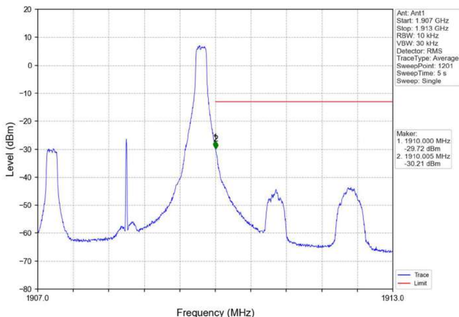
Band2_3MHz_QPSK_HCH_1908.5MHz_RB_1_14_NTNV
