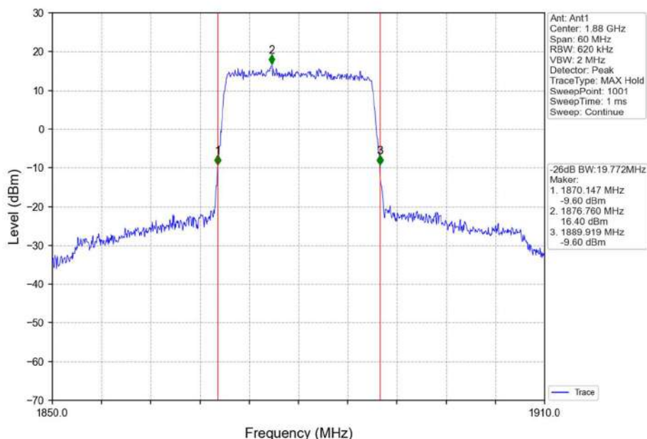
Band2_20MHz_QPSK_MCH_1880MHz_RB_100_0_NTNV
