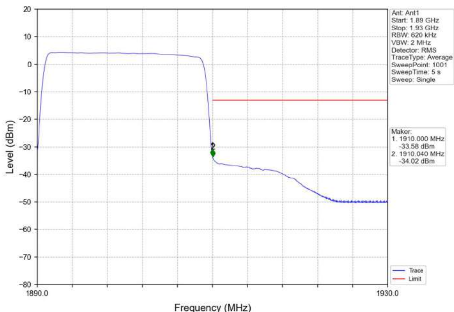
Band2_20MHz_16QAM_HCH_1900MHz_RB_100_0_NTNV
