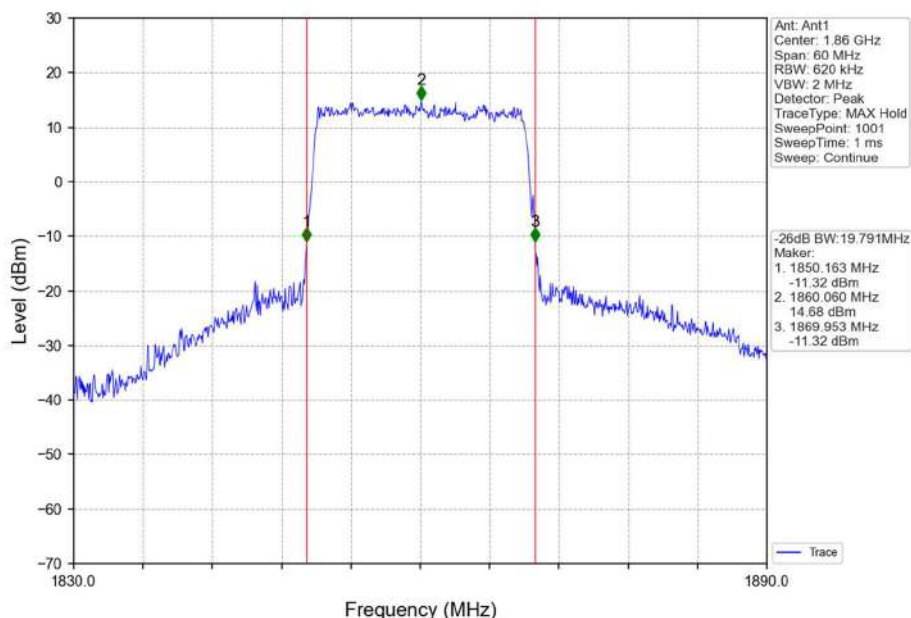
Band2_20MHz_16QAM_LCH_1860MHz_RB_100_0_NTNV
