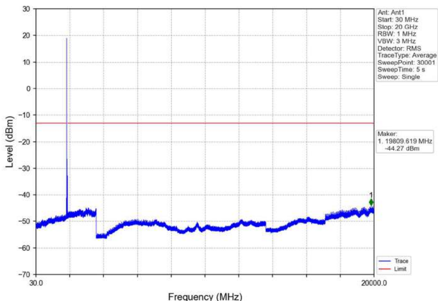
Band2_20MHz_16QAM_LCH_1860MHz_RB_1_0_NTNV
