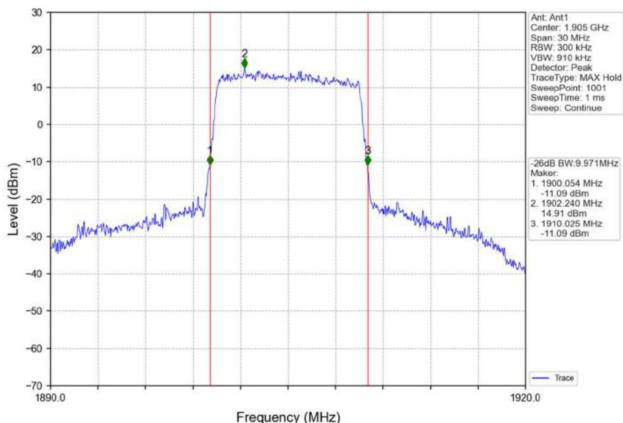
Band2_10MHz_16QAM_HCH_1905MHz_RB_50_0_NTNV
