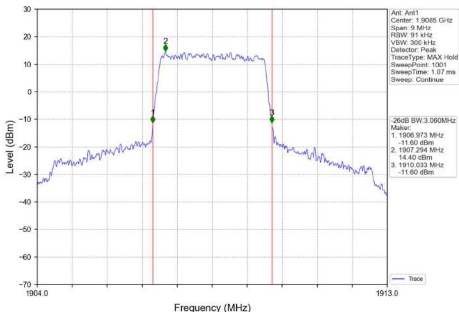
Band2_3MHz_QPSK_HCH_1908.5MHz_RB_15_0_NTNV
