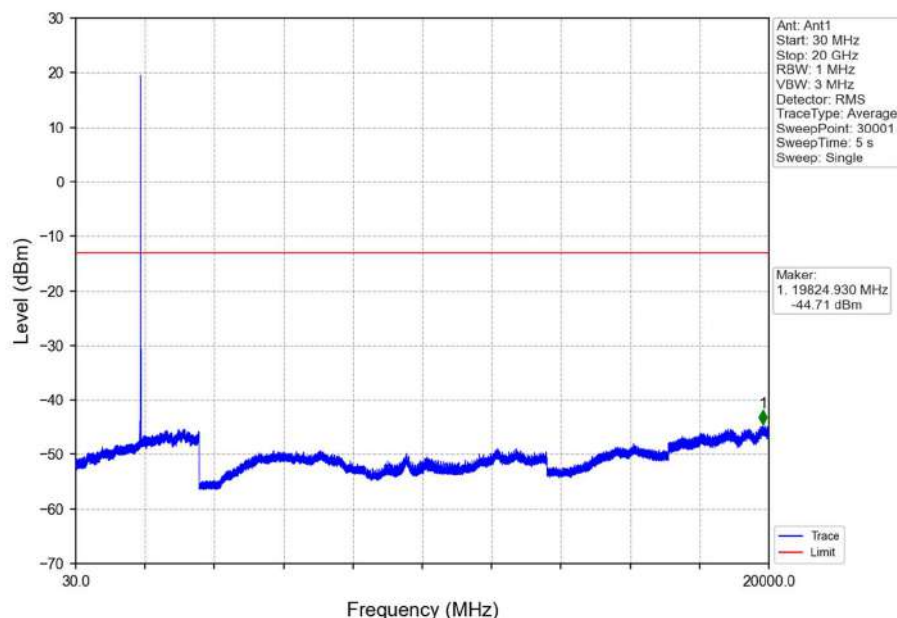
Band2_10MHz_QPSK_HCH_1905MHz_RB_1_0_NTNV
