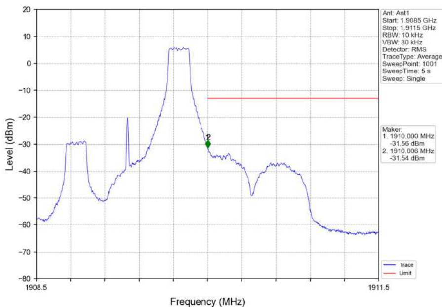
Band2 1.4MHz 16QAM HCH 1909.3MHz RB 1 5 NTNV
