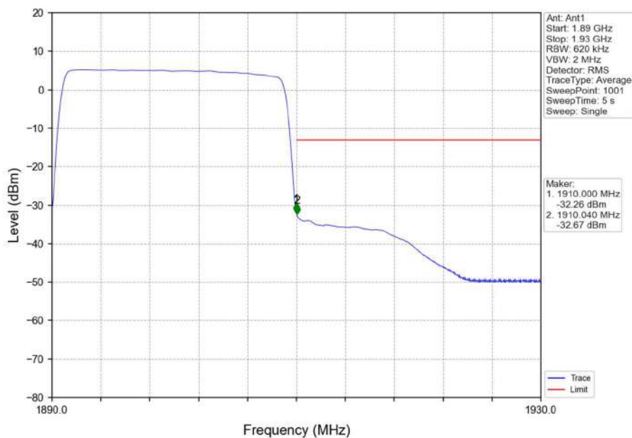
Band2_20MHz_QPSK_HCH_1900MHz_RB_100_0_NTNV
