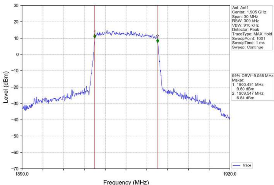
Band2_10MHz_16QAM_HCH_1905MHz_RB_50_0_NTNV
