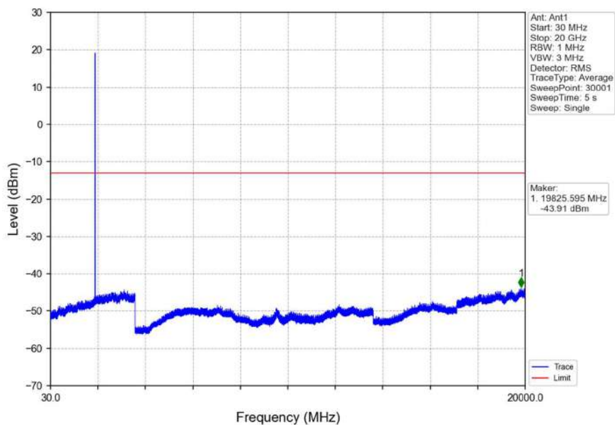
Band2_3MHz_QPSK_HCH_1908.5MHz_RB_1_0_NTNV
