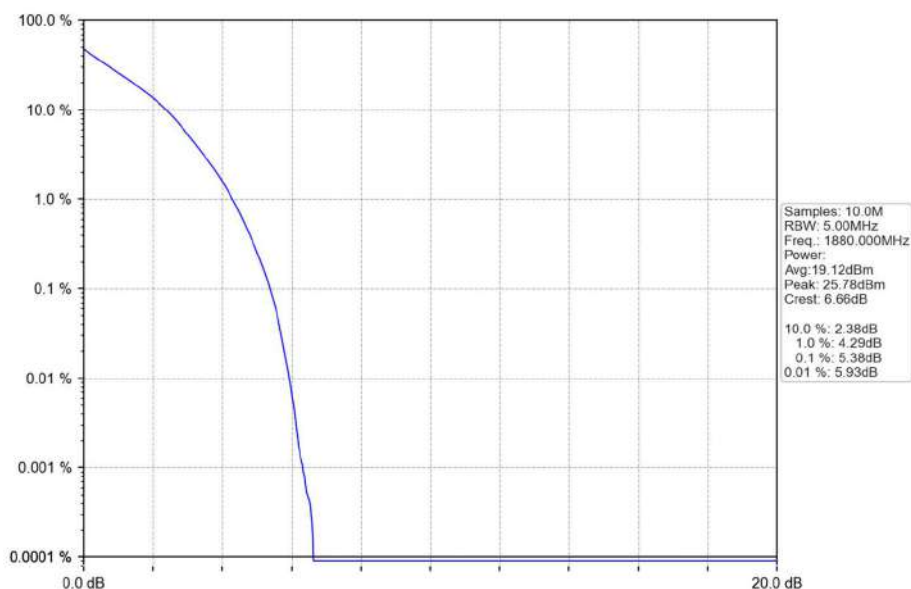
Band2_5MHz_QPSK_MCH_1880MHz_RB_25_0_NTNV
