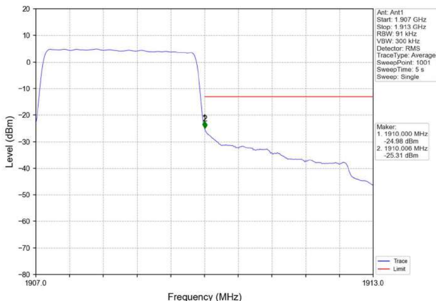
Band2_3MHz_QPSK_HCH_1908.5MHz_RB_15_0_NTNV
