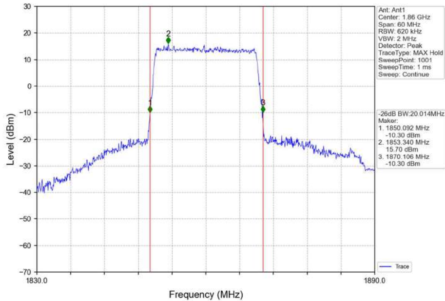
Band2_20MHz_QPSK_LCH_1860MHz_RB_100_0_NTNV
