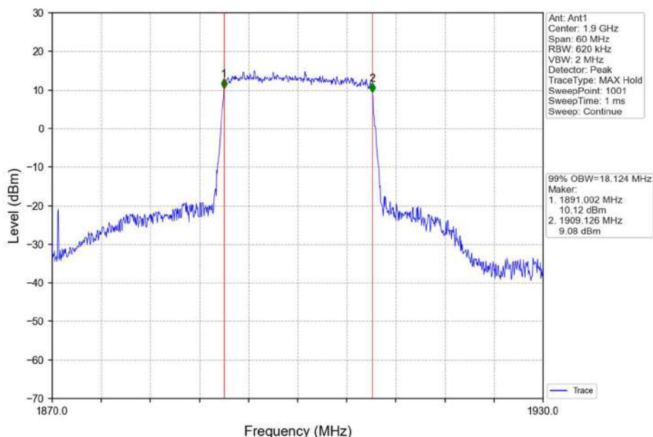
Band2_20MHz_16QAM_HCH_1900MHz_RB_100_0_NTNV
