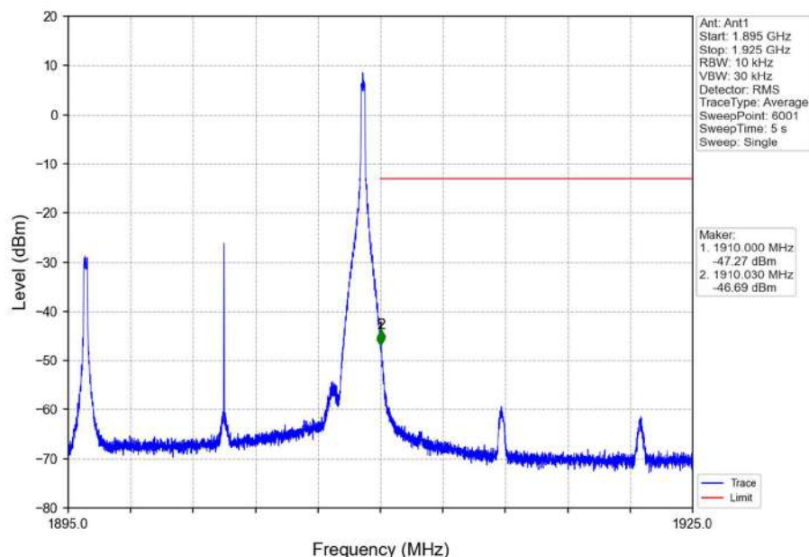
Band2_15MHz_16QAM_HCH_1902.5MHz_RB_1_74_NTNV
