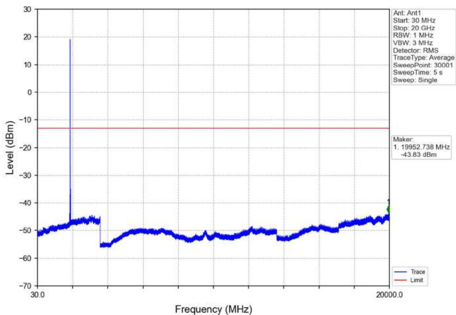
Band2_20MHz_16QAM_HCH_1900MHz_RB_1_0_NTNV
