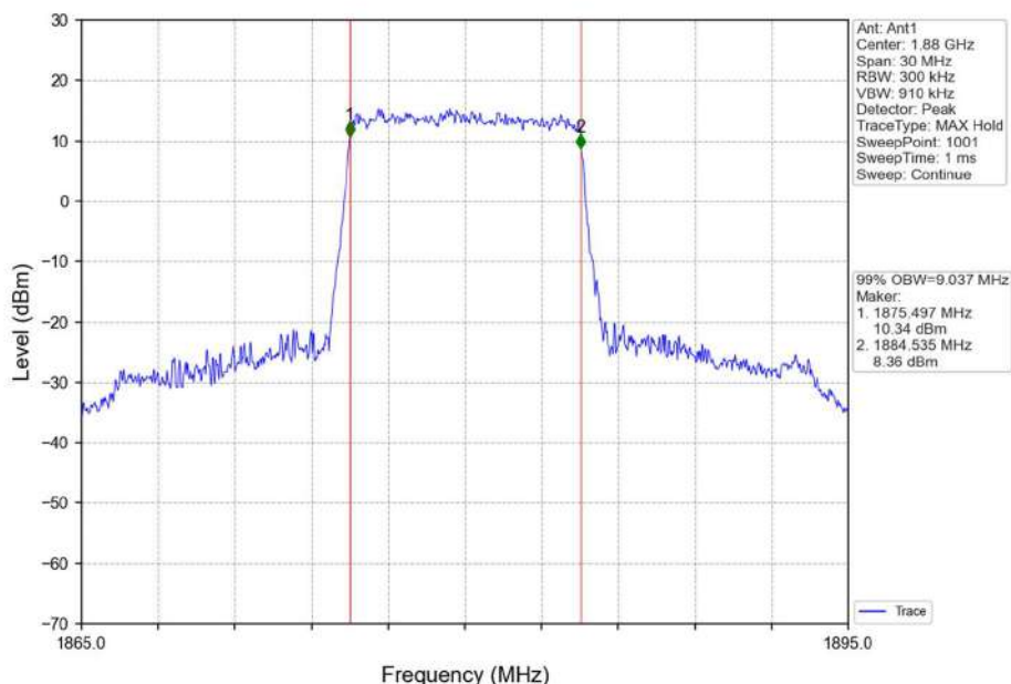
Band2_10MHz_QPSK_MCH_1880MHz_RB_50_0_NTNV
