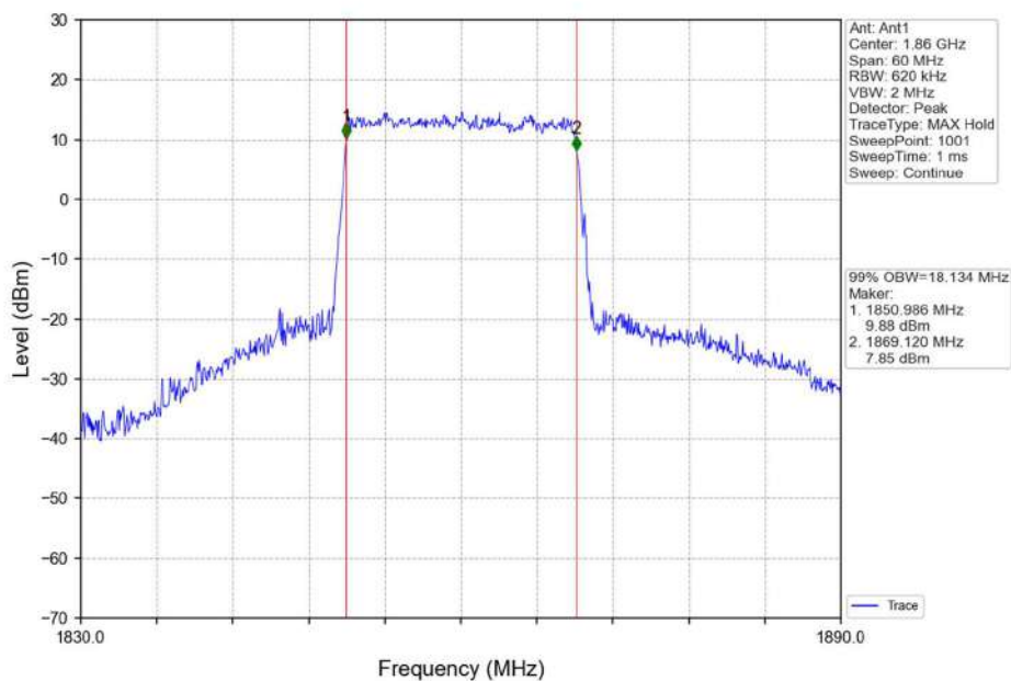
Band2_20MHz_16QAM_LCH_1860MHz_RB_100_0_NTNV
