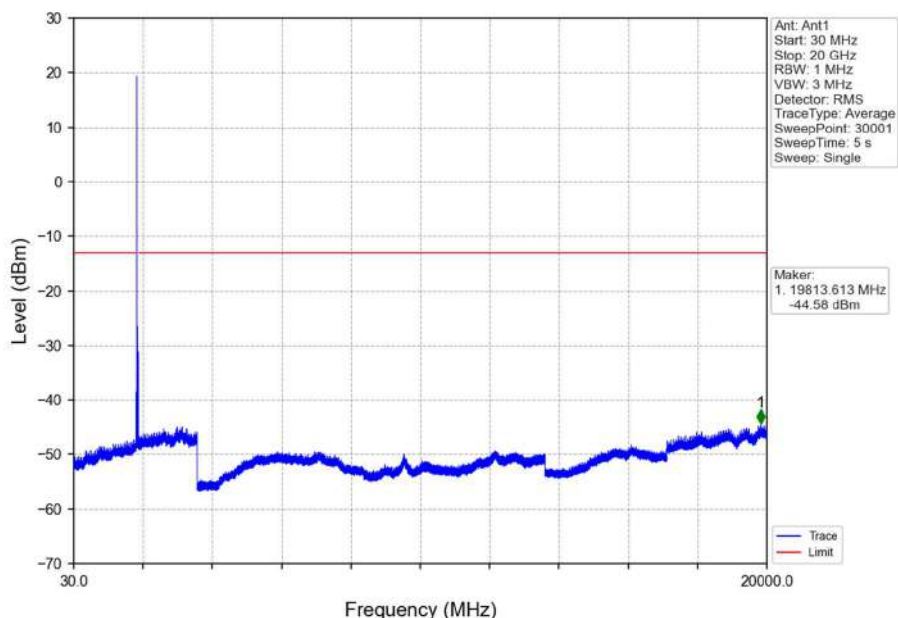
Band2_20MHz_QPSK_LCH_1860MHz_RB_1_0_NTNV
