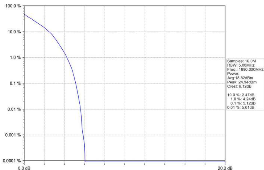
Band2_3MHz_QPSK_MCH_1880MHz_RB_15_0_NTNV
