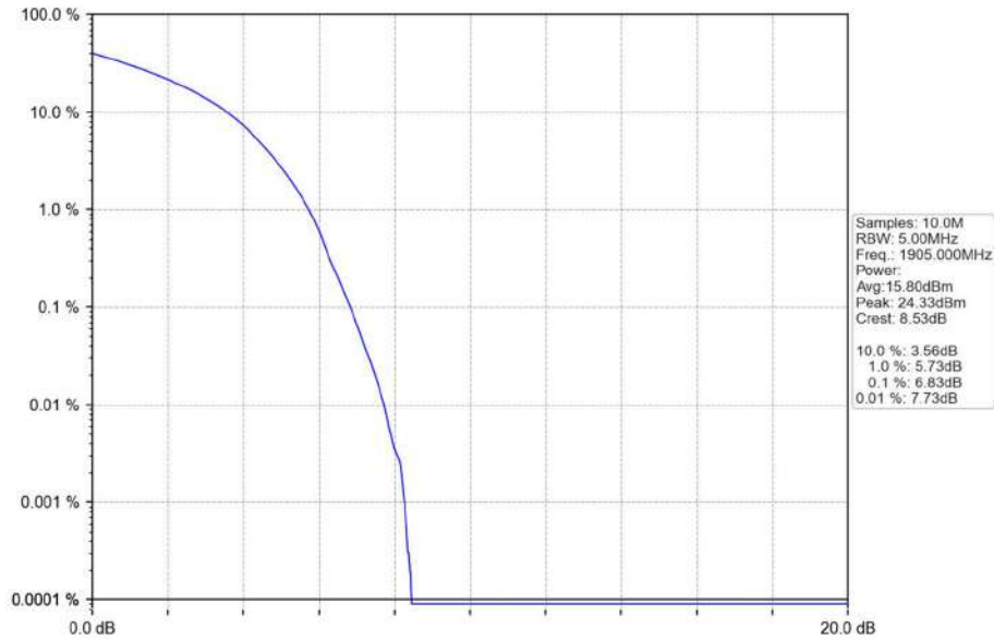
Band2_10MHz_16QAM_HCH_1905MHz_RB_50_0_NTNV
