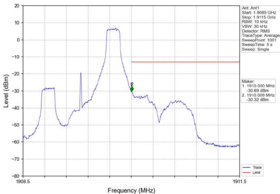
Band2_1.4MHz_QPSK_HCH_1909.3MHz_RB_1_5_NTNV
