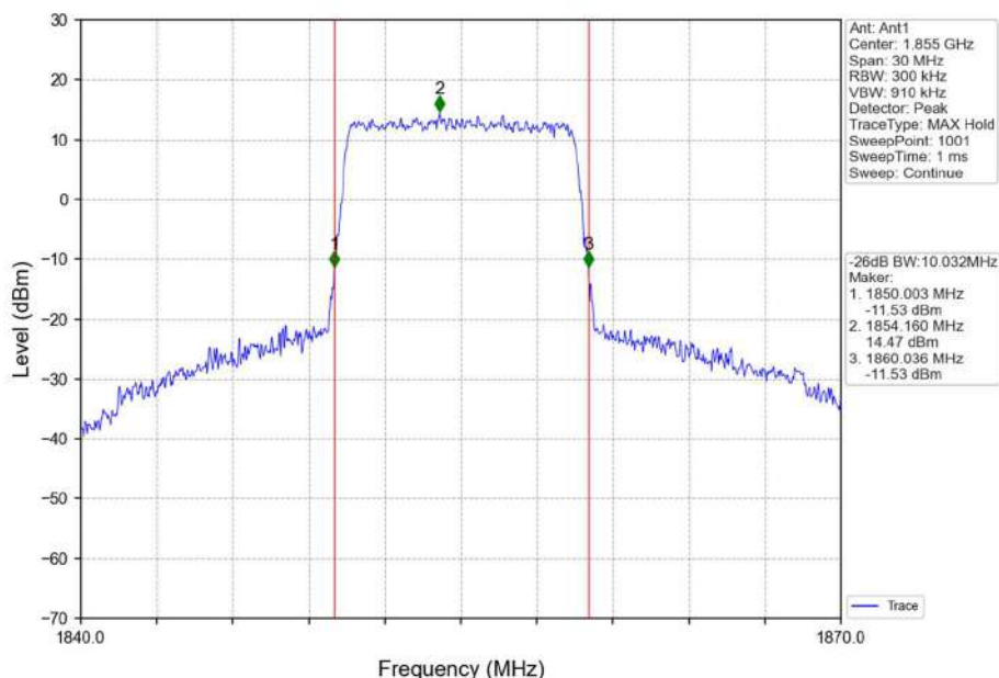
Band2_10MHz_16QAM_LCH_1855MHz_RB_50_0_NTNV
