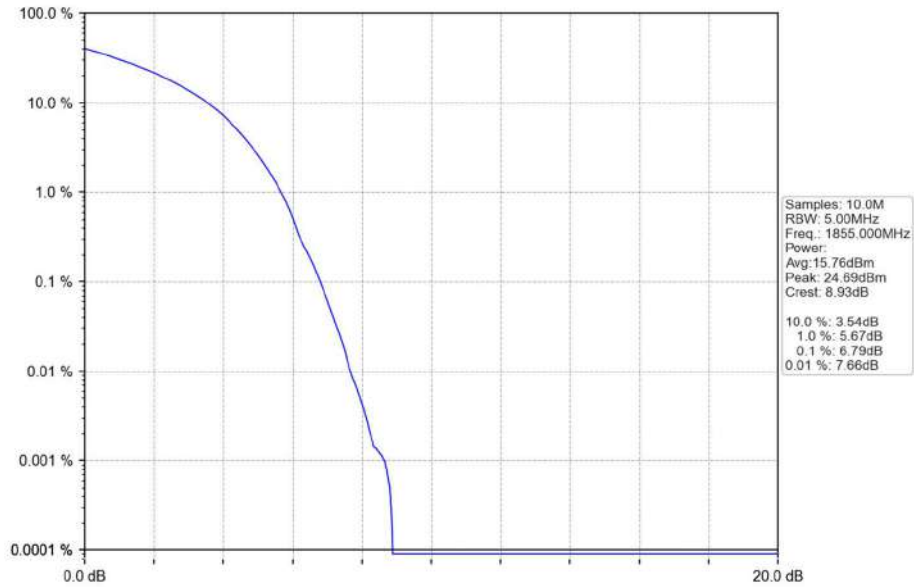
Band2_10MHz_16QAM_LCH_1855MHz_RB_50_0_NTNV
