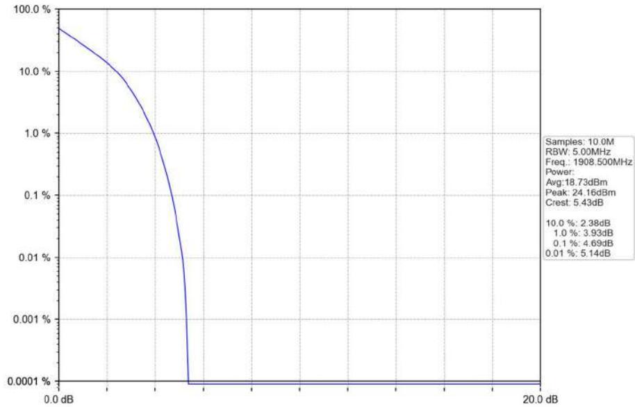
Band2_3MHz_QPSK_HCH_1908.5MHz_RB_15_0_NTNV
