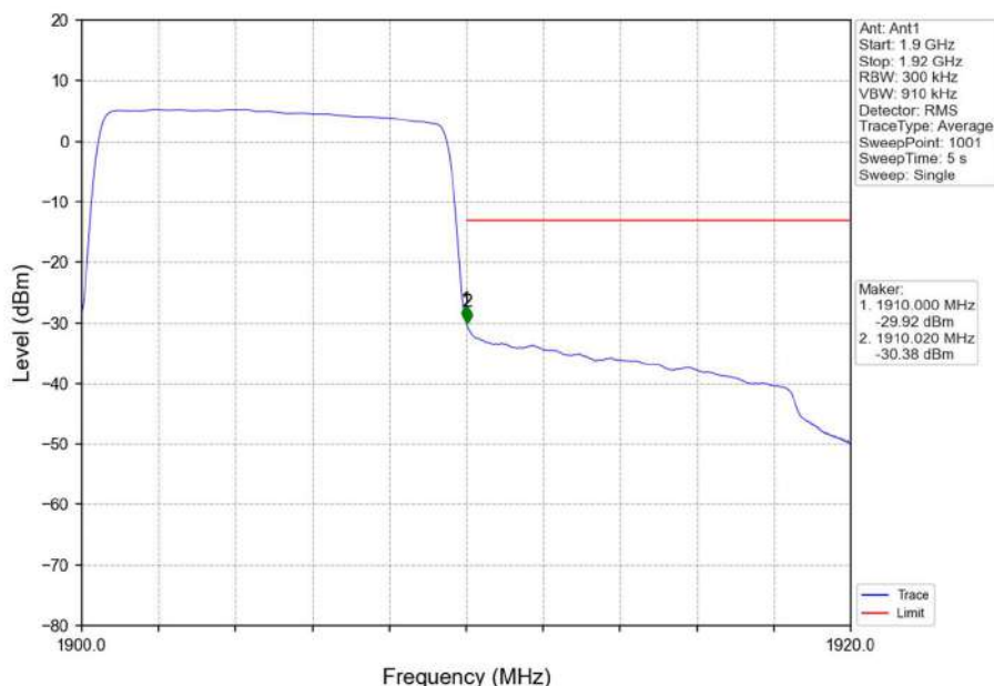
Band2_10MHz_QPSK_HCH_1905MHz_RB_50_0_NTNV
