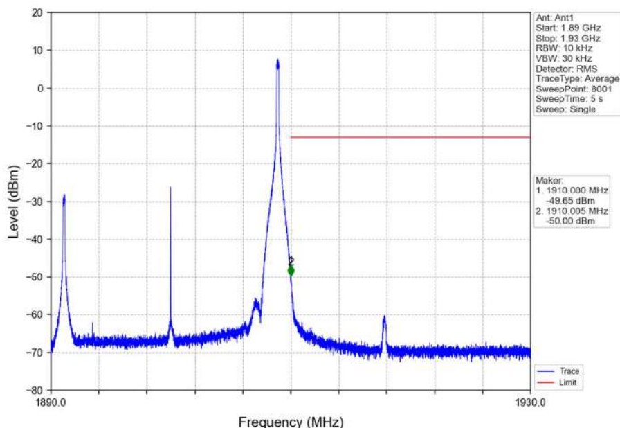
Band2_20MHz_16QAM_HCH_1900MHz_RB_1_99_NTNV
