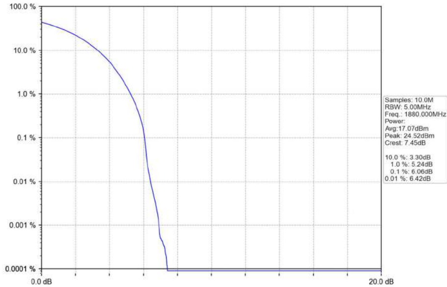
Band2_10MHz_QPSK_MCH_1880MHz_RB_50_0_NTNV
