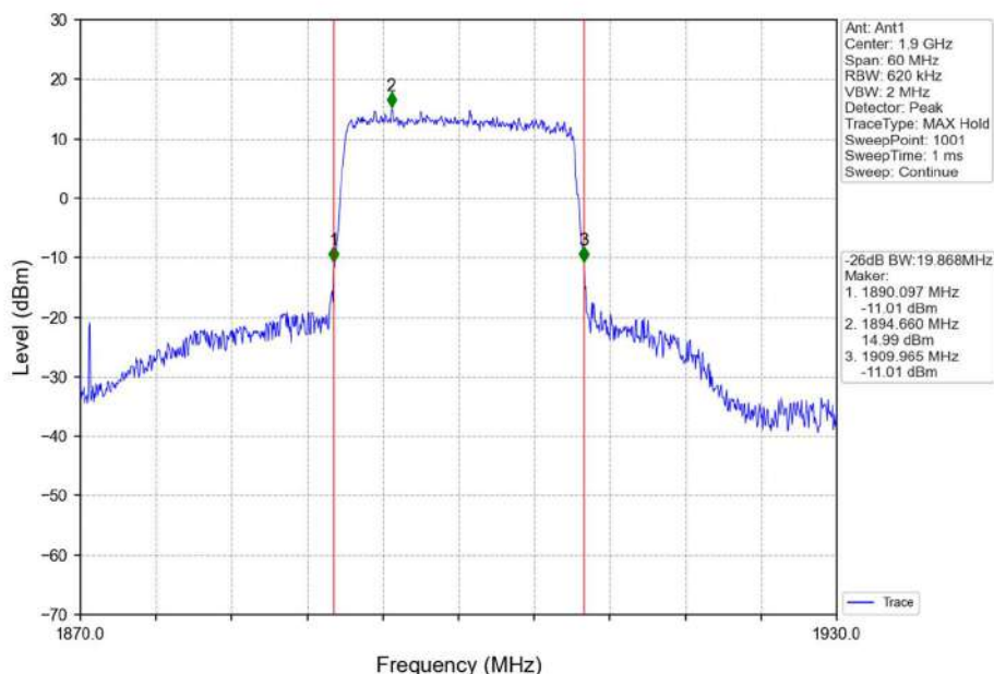
Band2_20MHz_16QAM_HCH_1900MHz_RB_100_0_NTNV
