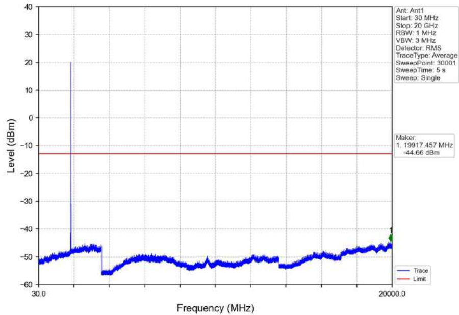
Band2_10MHz_QPSK_LCH_1855MHz_RB_1_0_NTNV
