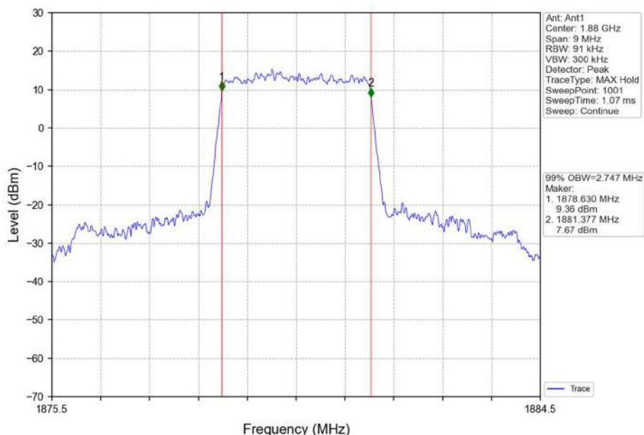
Band2_3MHz_QPSK_MCH_1880MHz_RB_15_0_NTNV
