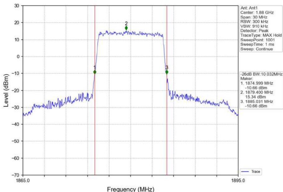
Band2_10MHz_QPSK_MCH_1880MHz_RB_50_0_NTNV
