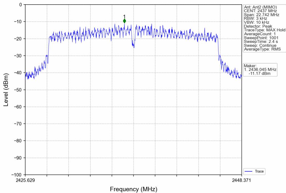
802.11ac(VHT20)_MCH_2437MHz_MIMO_NTNV
