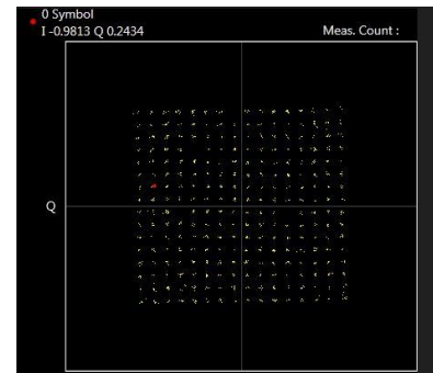
256QAM
