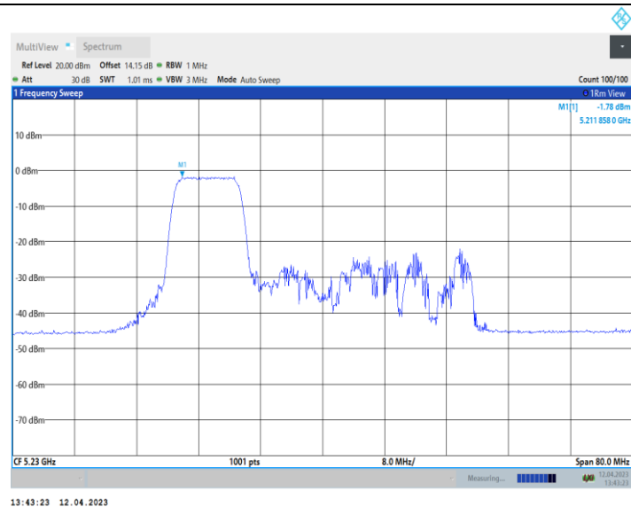
11AX40_Ant10_5230_242Tone_RU61
