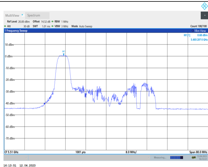
11AX40_Ant10_5510_242Tone_RU61
