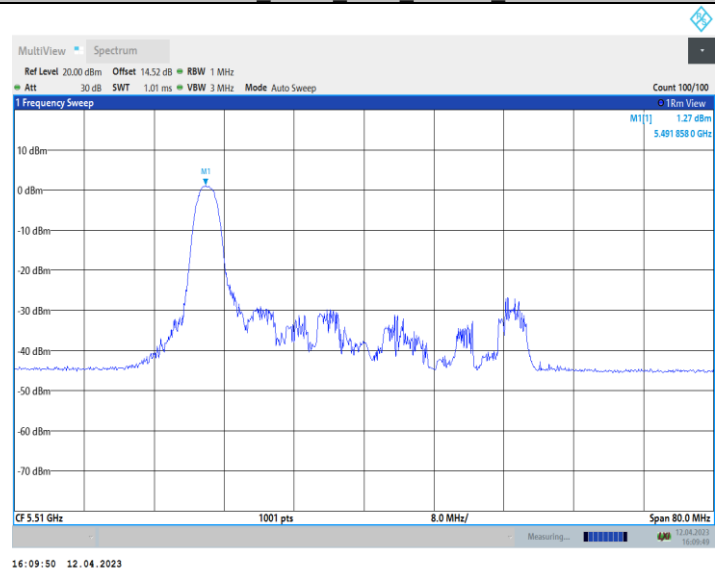
11AX40_Ant10_5510_52Tone_RU37
