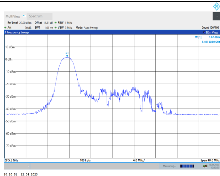
11AX20_Ant10_5500_52Tone_RU37
