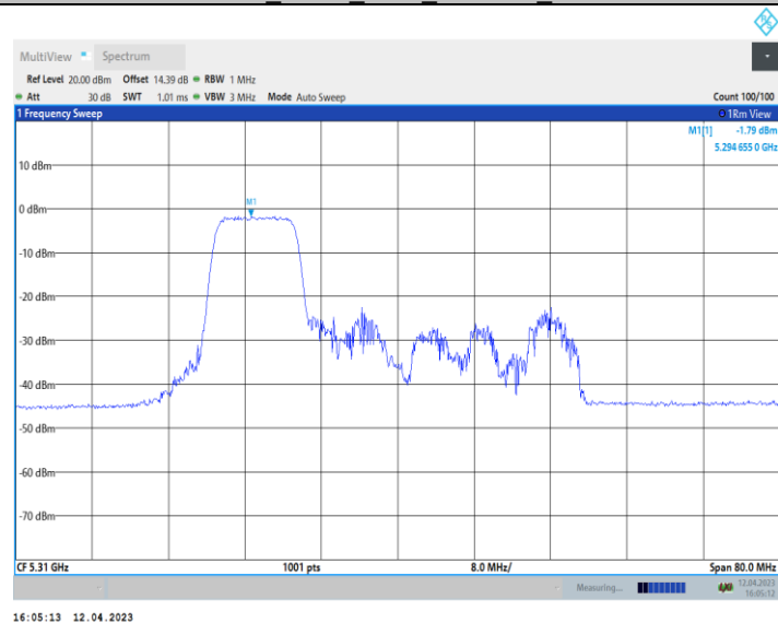
11AX40_Ant10_5310_242Tone_RU61
