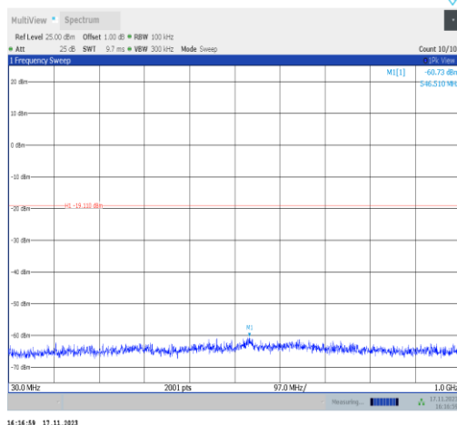
BLE_2M-Ant6-2404-30~1000-PASS
