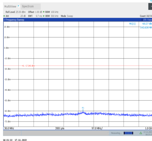
BLE_2M-Ant6-2440-30~1000-PASS
