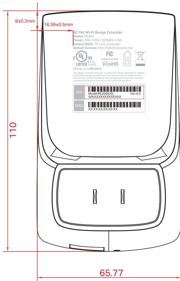
尺寸图
