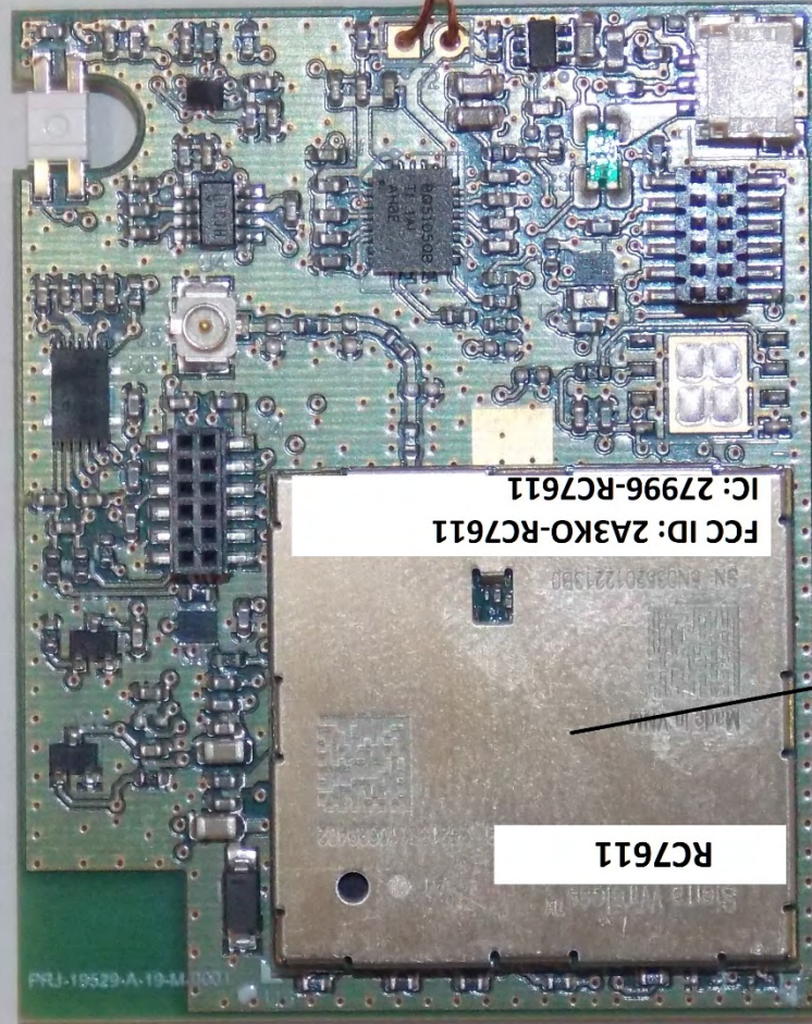
Cellular Module
