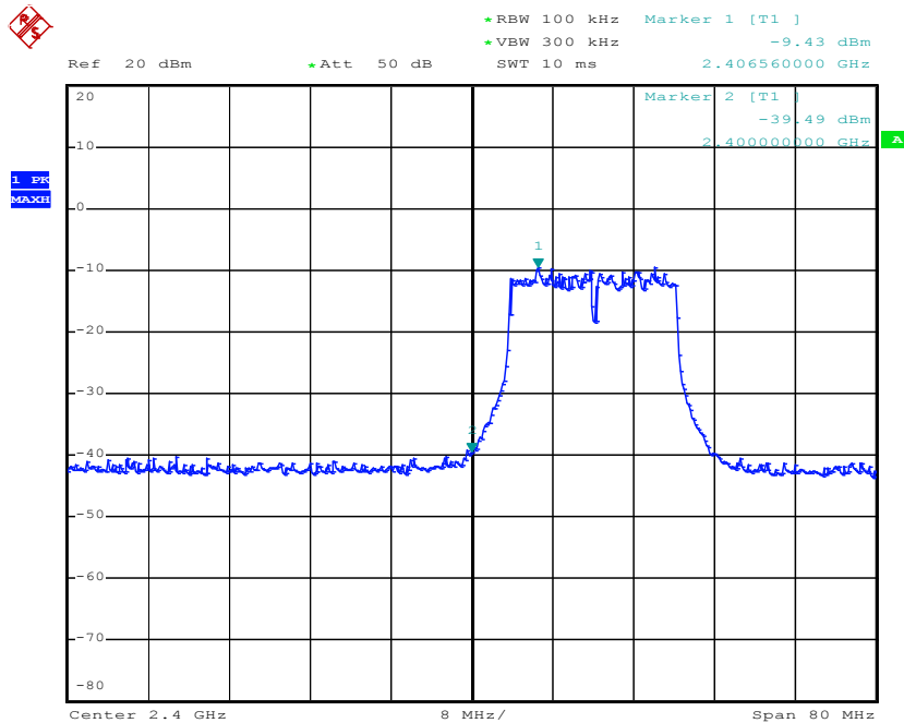
Figure 33: Lower Band Edge Conducted, 802.11 G AV and PK Detector
