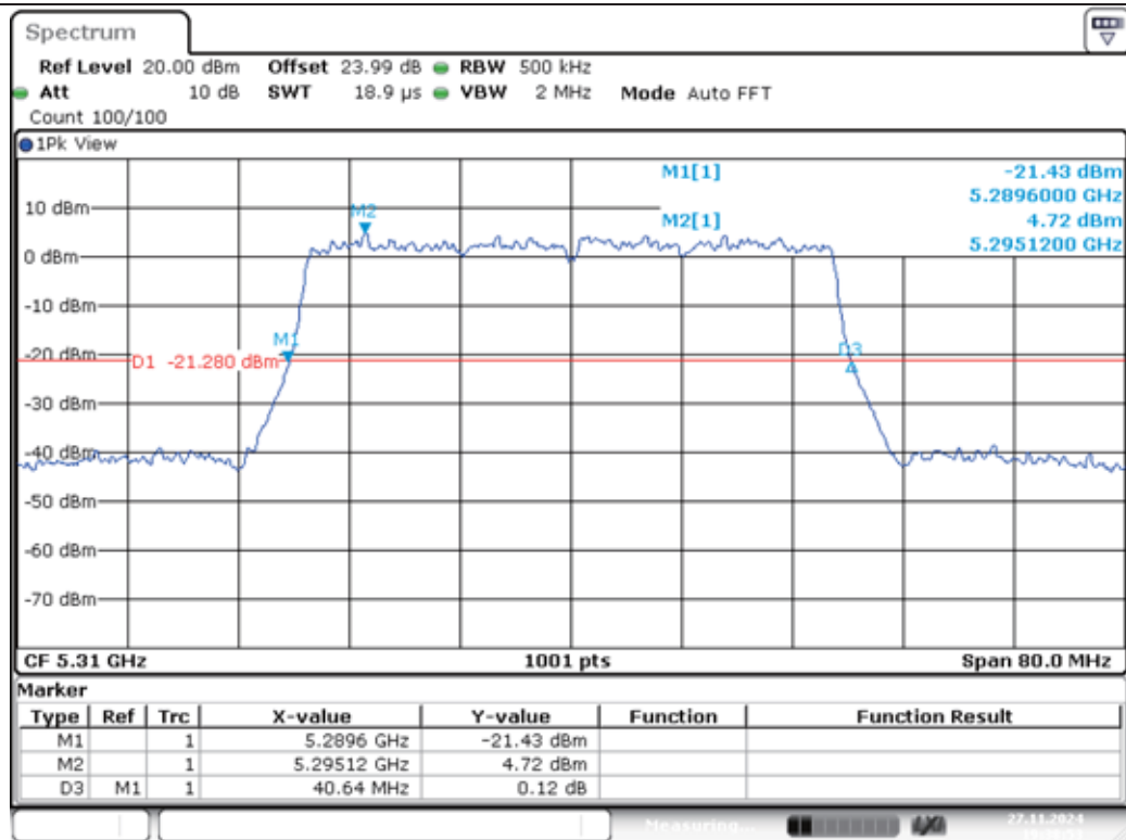
11AX40MIMO-Ant1-5310
