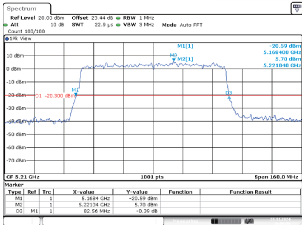
11AX80MIMO-Ant1-5210
