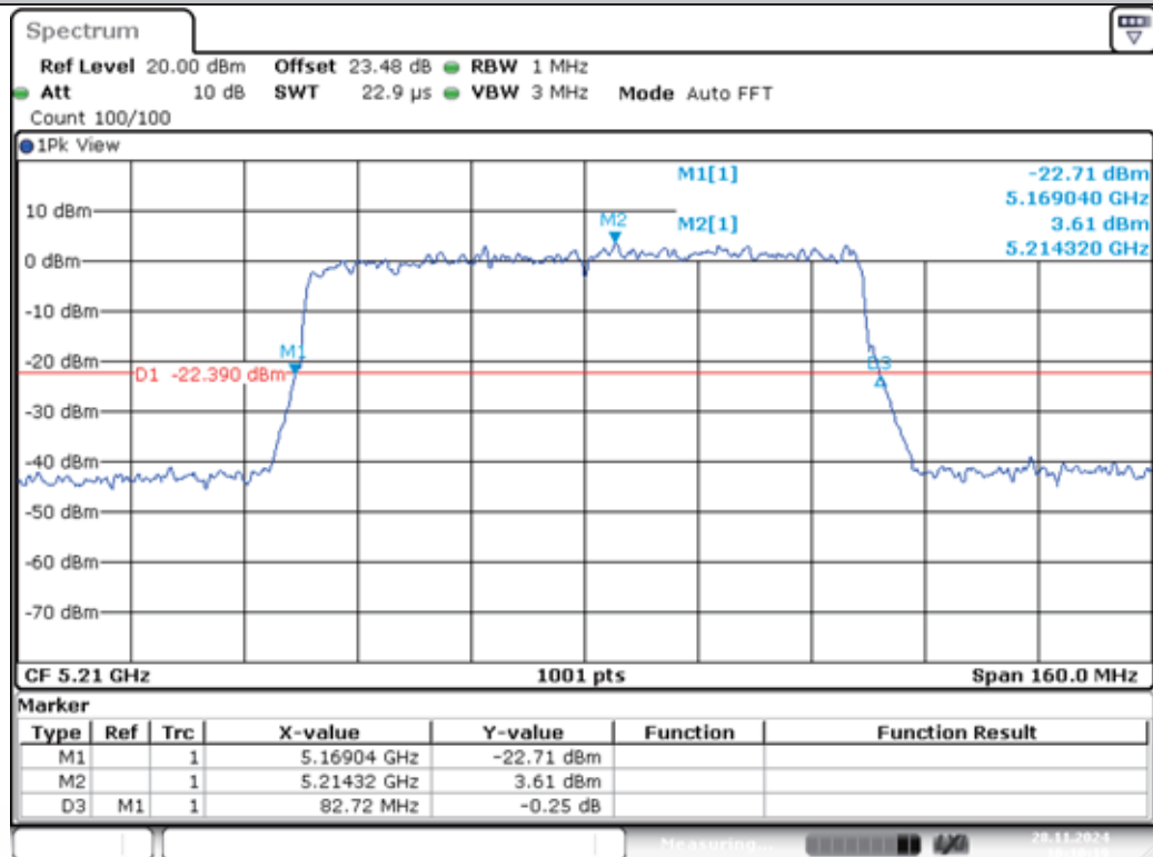
11AX80MIMO-Ant1-5210
