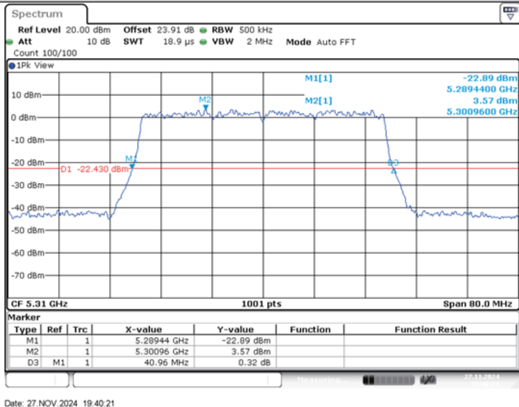
11AX40MIMO-Ant2-5310
