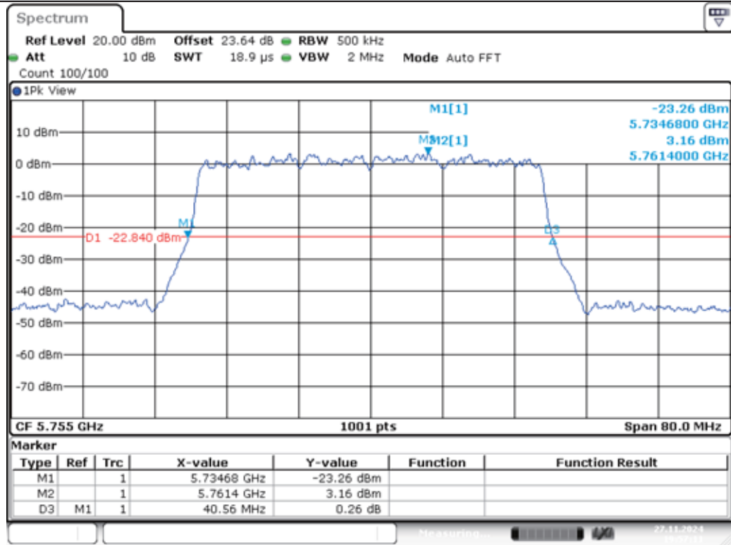
11AX40MIMO-Ant1-5755
