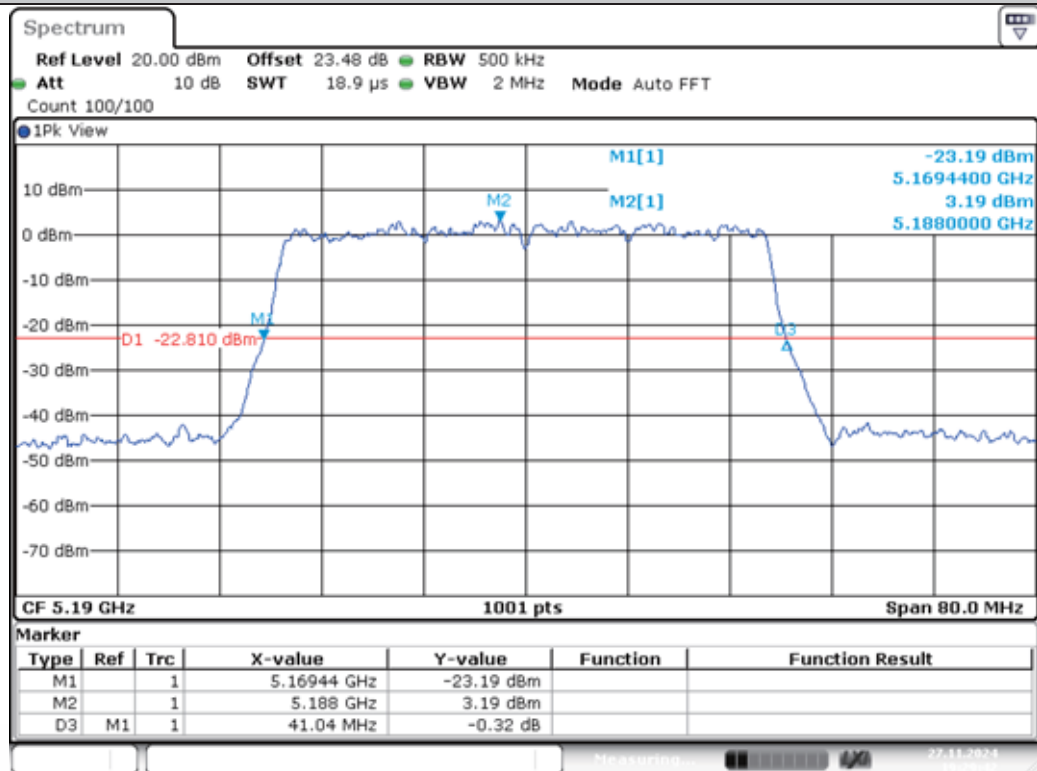
11AX40MIMO-Ant1-5190
