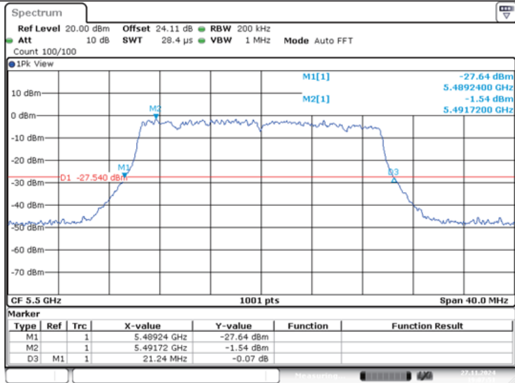
11AX20MIMO-Ant1-5500
