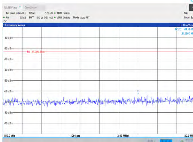
Band4-20MHz-QPSK-20050-1RB#0-Range2:0.15~30MHz
