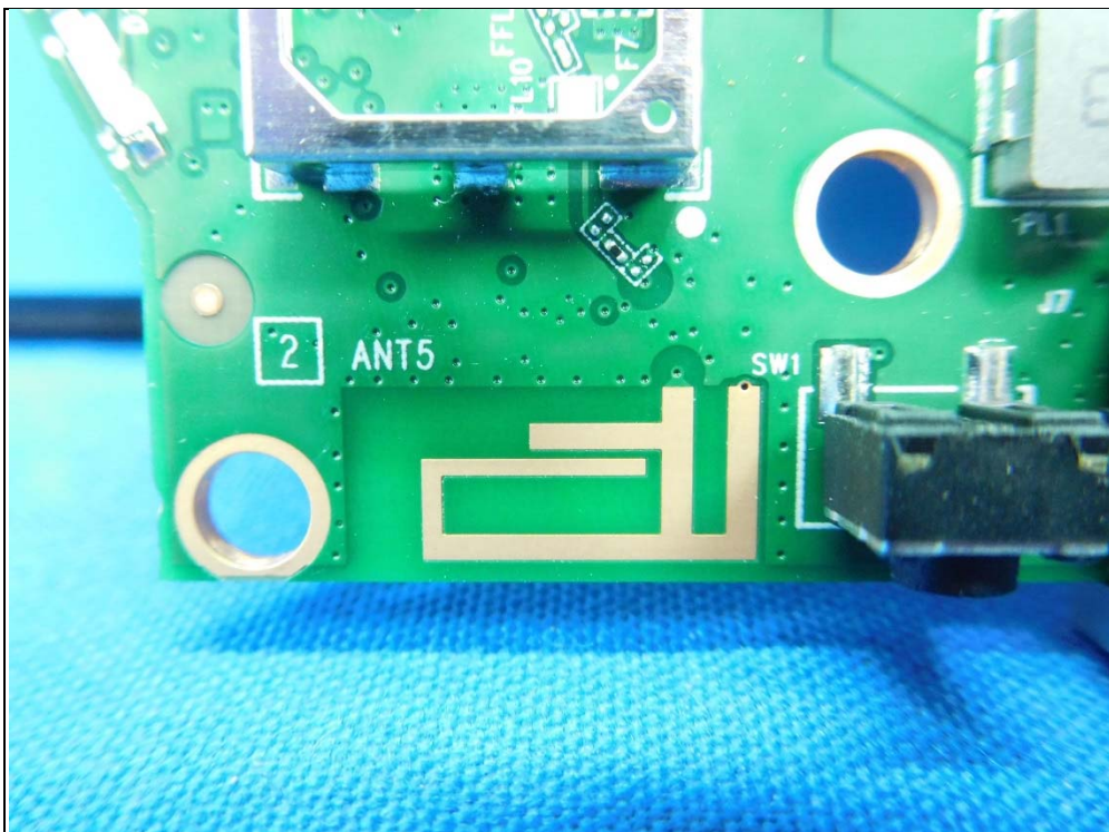
BT-LE Antenna
