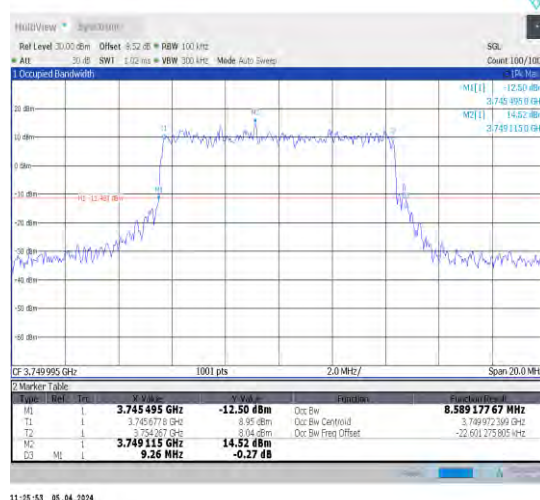
1-N78-3700-3800-N78-3700-380030-10-M-7-CP-16 QAM-Outer_Full-24@0-Ant1-8.589-9.260-≤10-PASS
