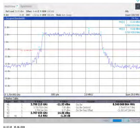
1-N78-3700-3800-N78-3700-380030-10-L-4-DFT-64 QAM-Outer_Full-24@0-Ant1-8.54-9.400-≤10-PASS
