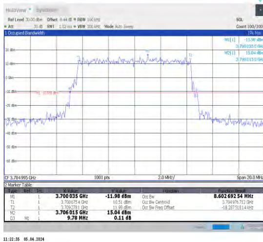
1-N78-3700-3800-N78-3700-380030-10-L-1-DFT-QP SK-Outer_Full-24@0-Ant1-8.603-9.780-≤10-PASS
