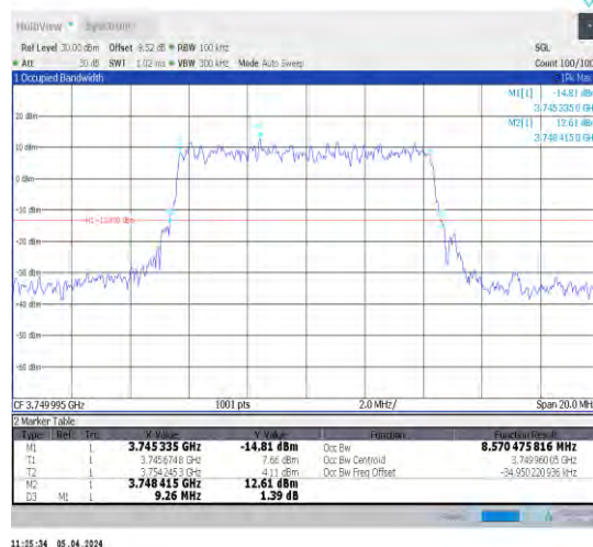
1-N78-3700-3800-N78-3700-380030-10-M-5-DFT-25 6QAM-Outer_Full-24@0-Ant1-8.57-9.260-≤10-PASS
