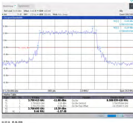
1-N78-3700-3800-N78-3700-380030-10-L-3-DFT-16 QAM-Outer_Full-24@0-Ant1-8.588-9.460-≤10-PASS
