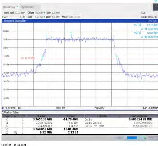
1-N78-3700-3800-N78-3700-380030-10-M-4-DFT-64 QAM-Outer_Full-24@0-Ant1-8.606-9.520-≤10-PASS
