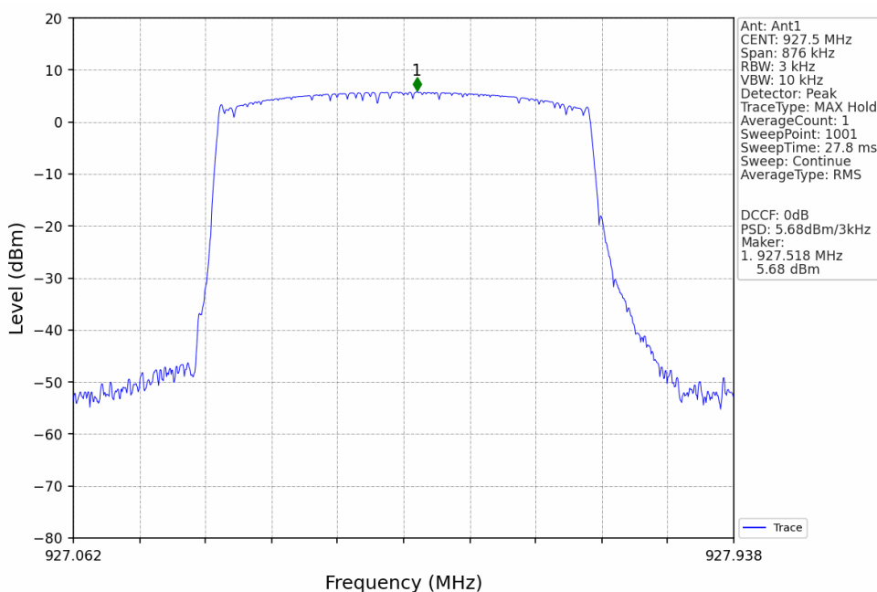
SF12_HCH_927.5MHz_Ant1_NTNV
