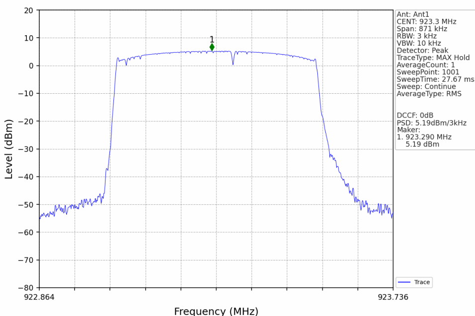
SF12_LCH_923.3MHz_Ant1_NTNV
