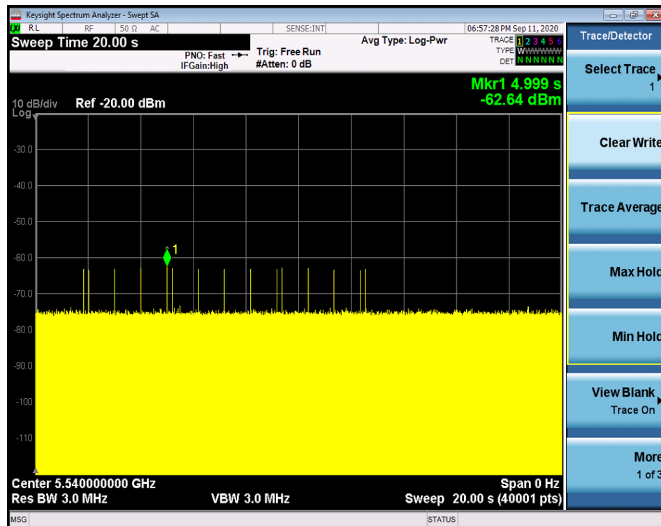
Radarsignal 5
