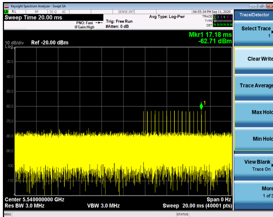
Radarsignal 3
