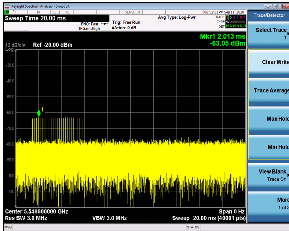
Radarsignal 3
