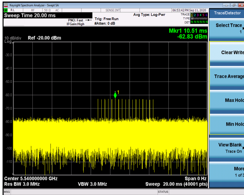
Radarsignal 5
