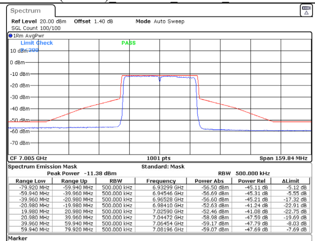
802.11ax (40MHz) 7005MHz Chain D NSS-2
