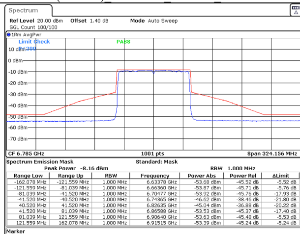
802.11ax (80MHz) 6785MHz Chain C NSS-2
