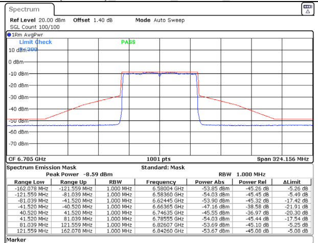
802.11ax (80MHz) 6705MHz Chain D NSS-2
