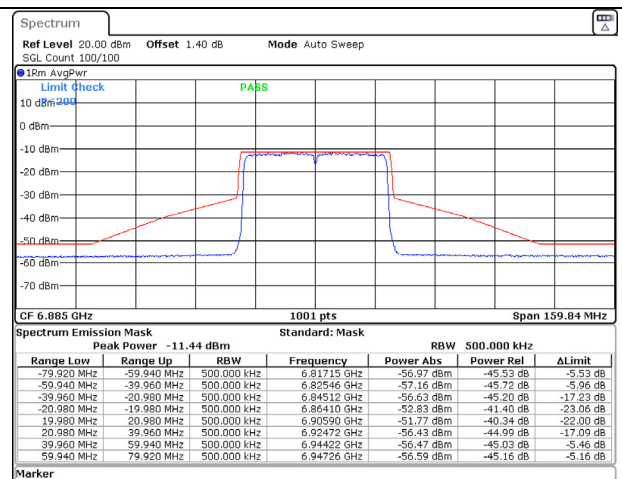
802.11ax (40MHz) 6885MHz Chain D NSS-2
