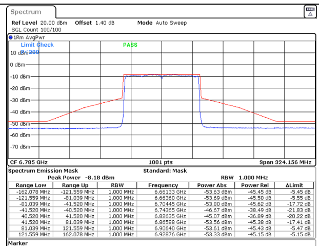
802.11ax (80MHz) 6785MHz Chain B NSS-2
