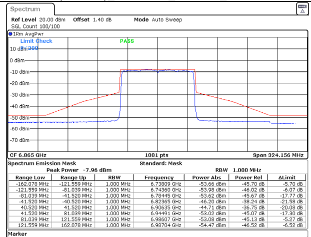
802.11ax (80MHz) 6865MHz Chain B NSS-2
