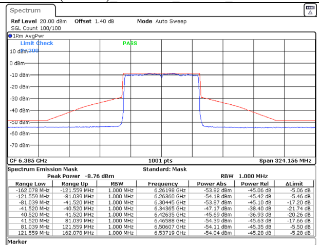
802.11ax (80MHz) 6385MHz Chain B NSS-2
