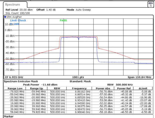
802.11ax (40MHz) 6925MHz Chain D NSS-2
