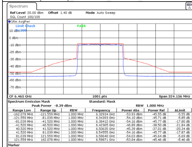
802.11ax (80MHz) 6465MHz Chain C NSS-2
