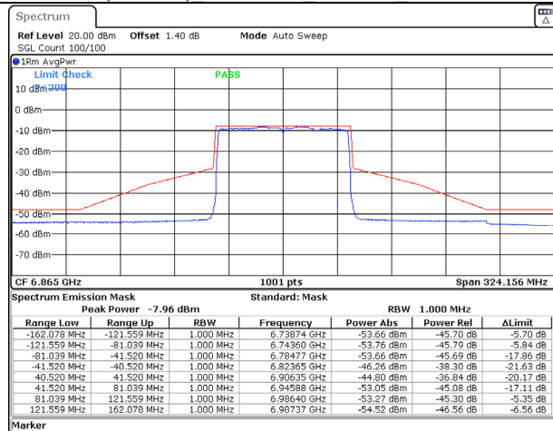
802.11ax (80MHz) 6865MHz Chain A NSS-2
