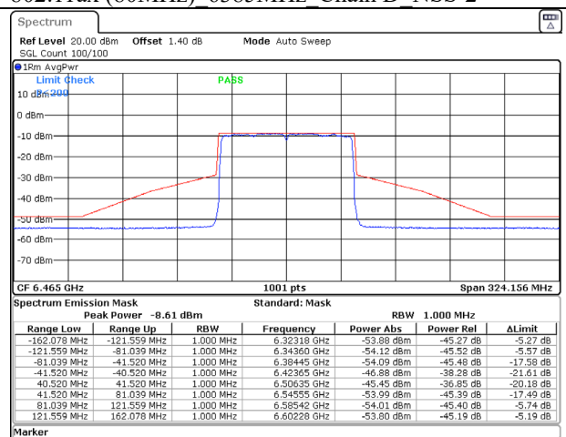
802.11ax (80MHz) 6465MHz Chain B NSS-2
