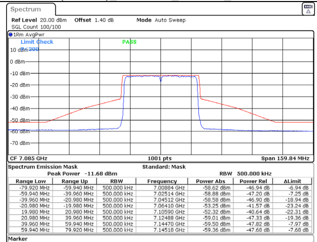
802.11ax (40MHz) 7085MHz Chain B NSS-2
