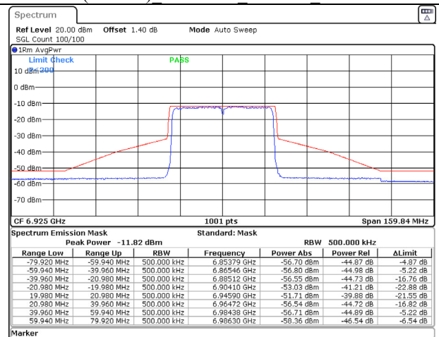
802.11ax (40MHz) 6925MHz Chain B NSS-2
