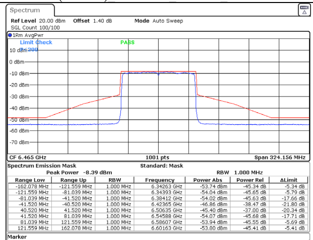
802.11ax (80MHz) 6465MHz Chain D NSS-2
