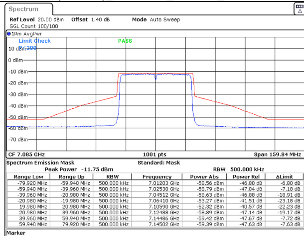
802.11ax (40MHz) 7085MHz Chain A NSS-2
