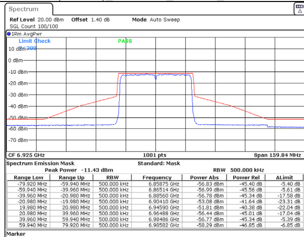
802.11ax (40MHz) 6925MHz Chain C NSS-2
