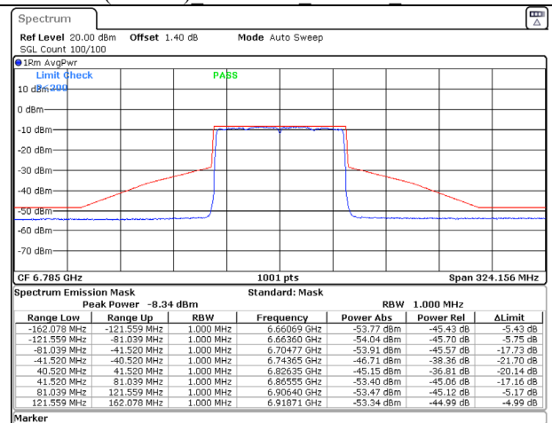
802.11ax (80MHz) 6785MHz Chain D NSS-2
