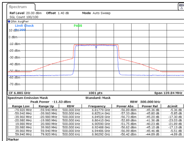
802.11ax (40MHz) 6885MHz Chain C NSS-2
