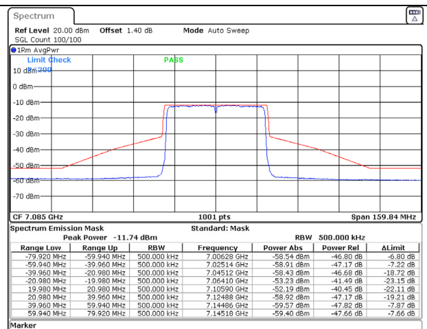
802.11ax (40MHz) 7085MHz Chain D NSS-2
