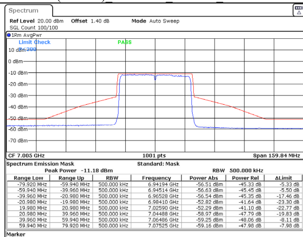
802.11ax (40MHz) 7005MHz Chain C NSS-2
