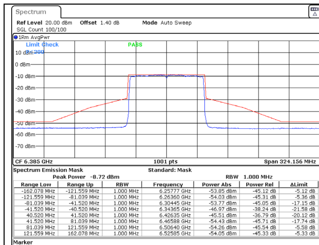
802.11ax (80MHz) 6385MHz Chain C NSS-2
