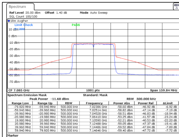
802.11ax (40MHz) 7085MHz Chain C NSS-2
