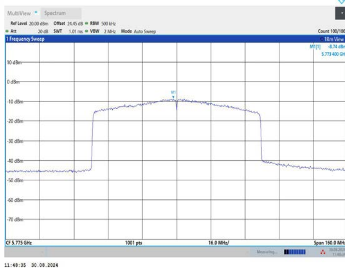
11BE80MIMO_Ant3_5775
