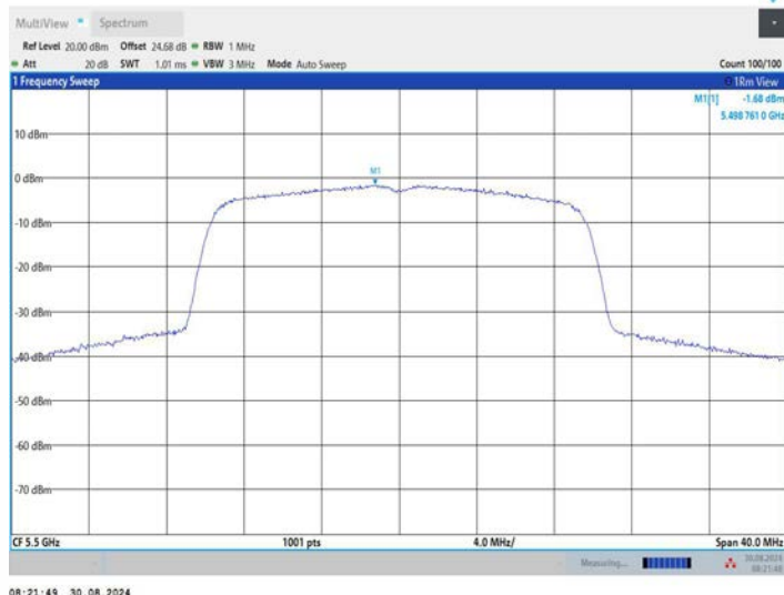
11BE20MIMO_Ant3_5500
