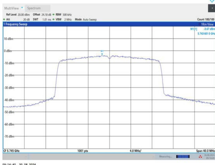
11BE20MIMO_Ant3_5745
