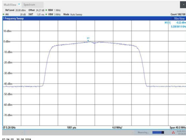
11BE20MIMO_Ant2_5260
