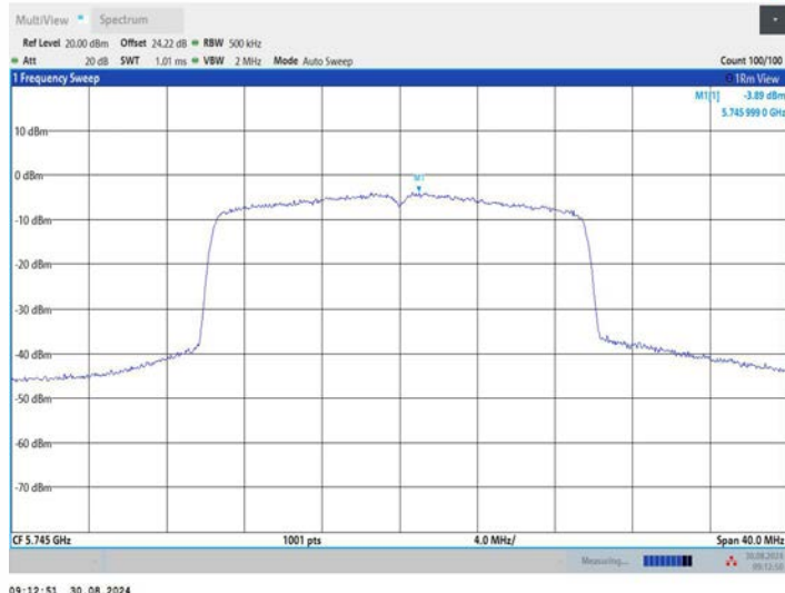
11BE20MIMO_Ant2_5745
