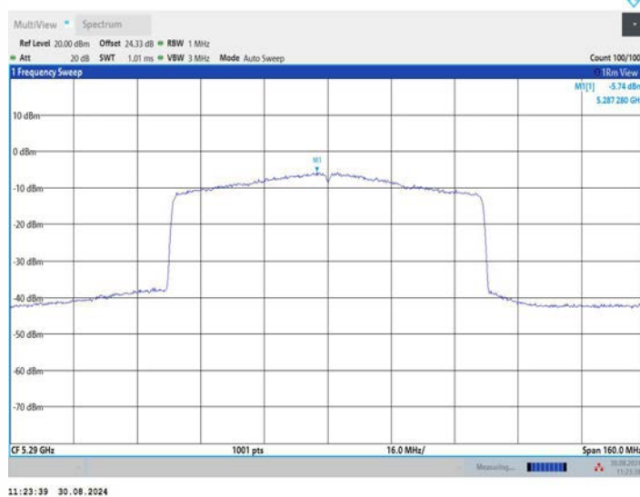
11BE80MIMO_Ant2_5290
