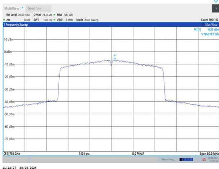
11BE40MIMO_Ant2_5795
