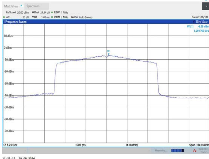
11BE80MIMO_Ant3_5290
