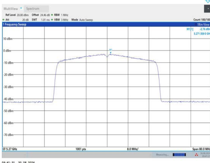
11BE40MIMO_Ant2_5270
