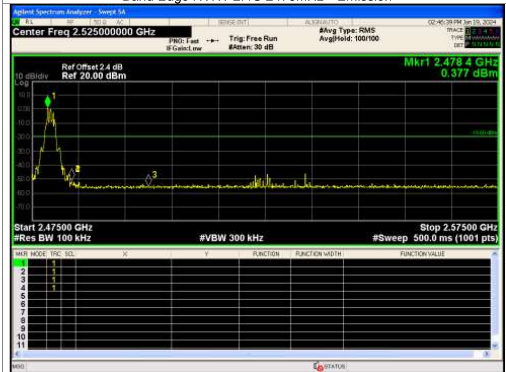
Band Edge NVNT 2.4G 2479MHz Emission
