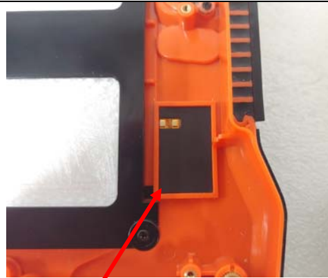
NFC Antenna
