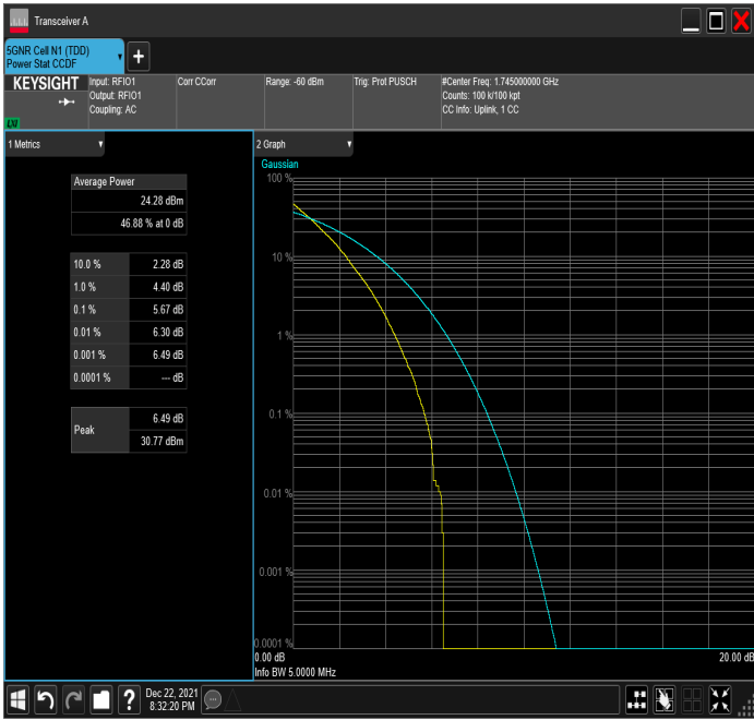
n66_5MHz_15kHz_1745MHz_DFT-s-OFDM QPSK_RB25@0
