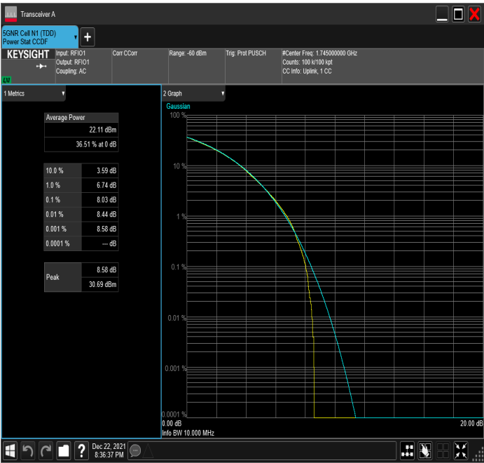
n66_10MHz_15kHz_1745MHz_CP-OFDM QPSK_RB50@0
