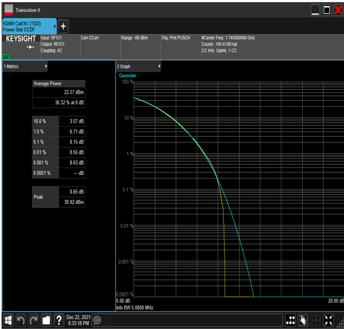
n66_5MHz_15kHz_1745MHz_CP-OFDM QPSK_RB25@0
