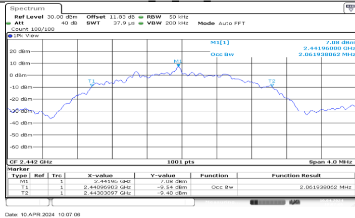
BLE 2M Ant1 2442
