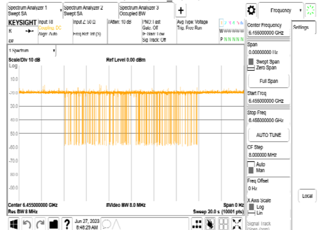
802.11be_20MHz_CF 6455MHz_Interference_6455MHz_-82.49dBm_Normal
