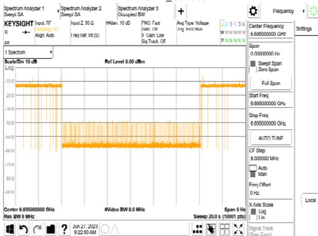
802.11be_20MHz_CF 6695MHz_Interference_6695MHz_-78.47dBm_Minimal
