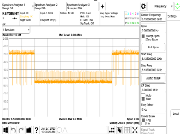
802.11be_20MHz_CF 6135MHz_Interference_6135MHz_-75.25dBm_Minimal
