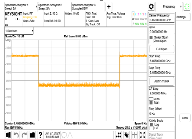
802.11be_20MHz_CF 6455MHz_Interference_6455MHz_-76.49dBm_Minimal
