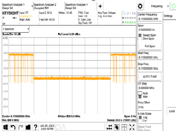
802.11be_320MHz_CF 6265MHz_Interference_6110MHz_ -73.48dBm_Minimal
