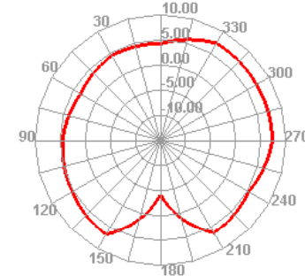
Bluetooth 39 TIS E2
