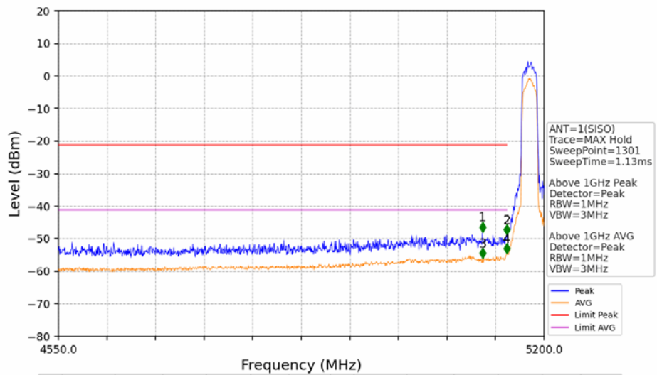
802.11ax(HEW20)_LCH_5180MHz_RU242_Left_Ant1_NTNV
