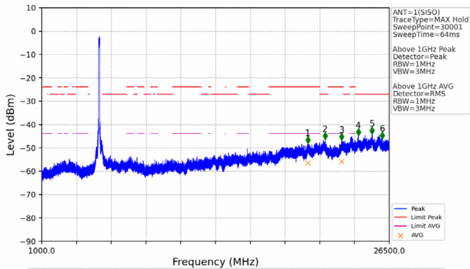
802.11ax(HEW80)_MCH_5210MHz_RU996_Left_Ant1_NTNV
