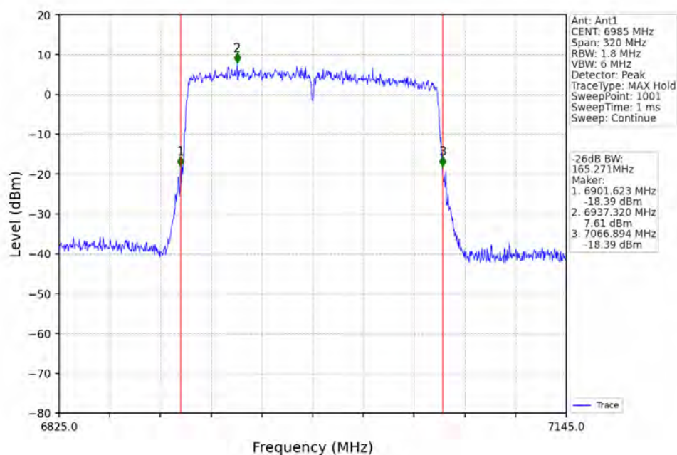
802.11ax(HEW160)_MCH_6985MHz_2xRU996_Left_Ant1_NTNV
