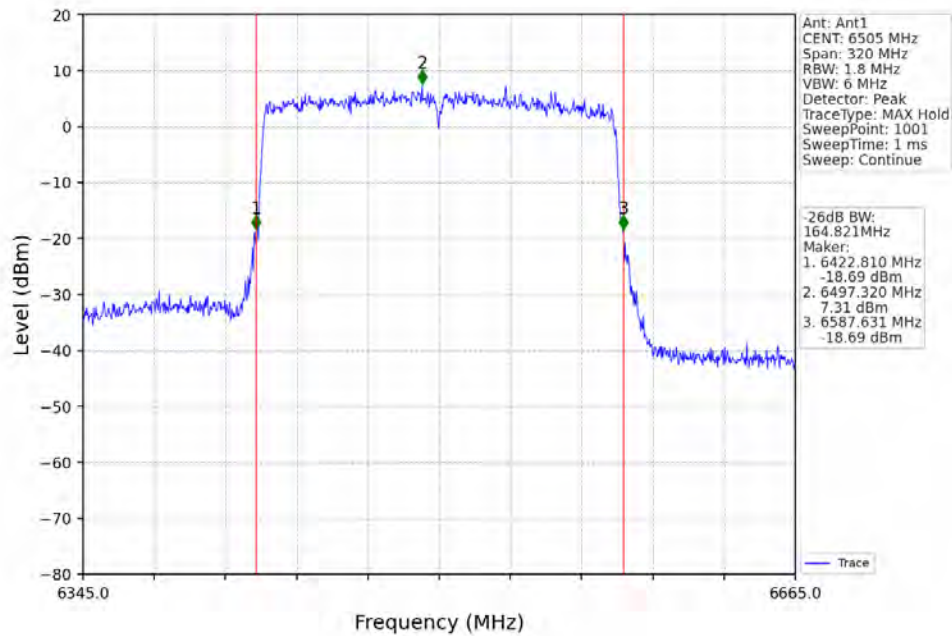
802.11ax(HEW160)_HCH_6505MHz_2xRU996_Left_Ant1_NTNV
