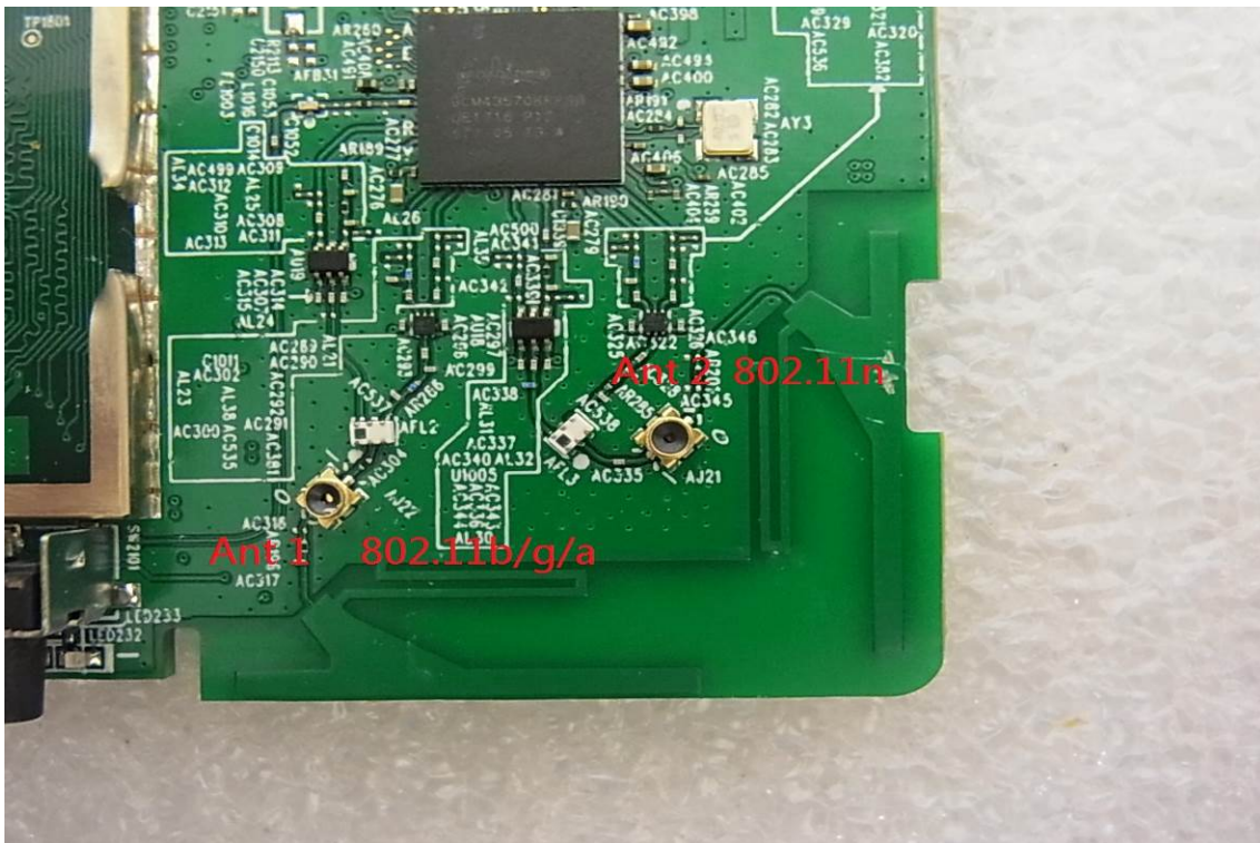
EUT 14
