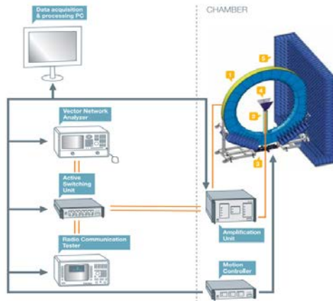
暗室系统配置图
