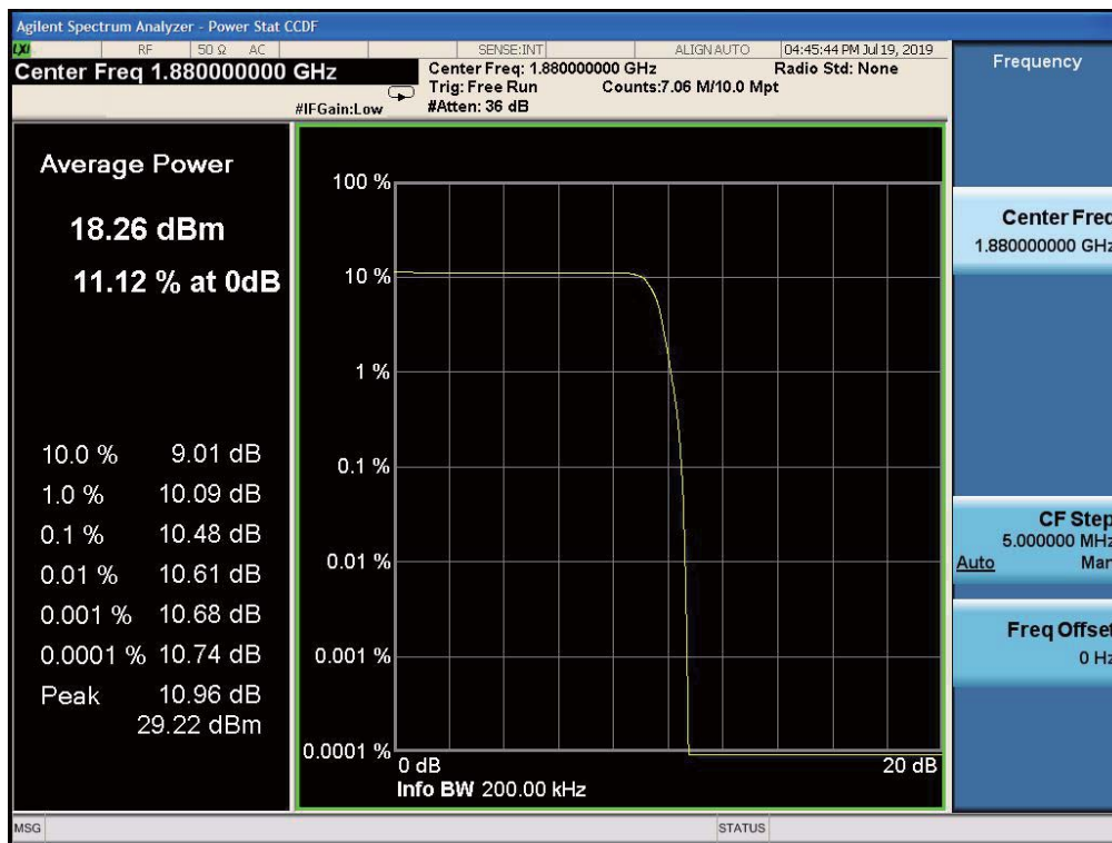
1880MHz-CH661-GMSK
