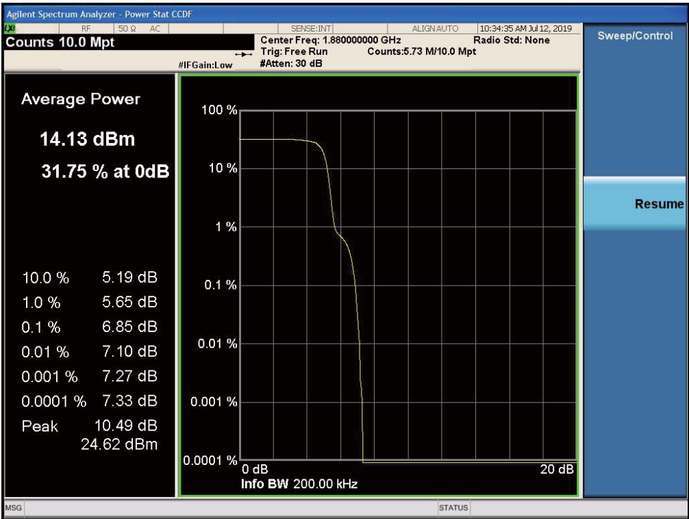
Band2-CH18900-1880MHz-BPSK
