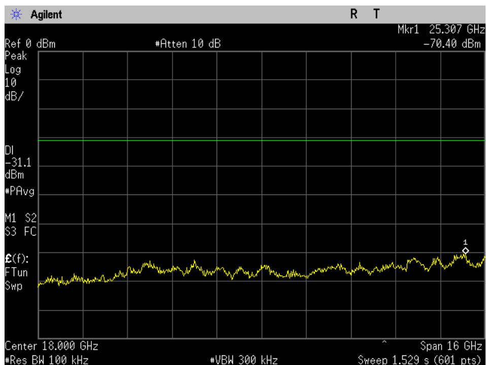
WIFI_Low Ch_2412MHz_20MHz BW_n-mode_-30dBc_10-26GHz_Port 1
