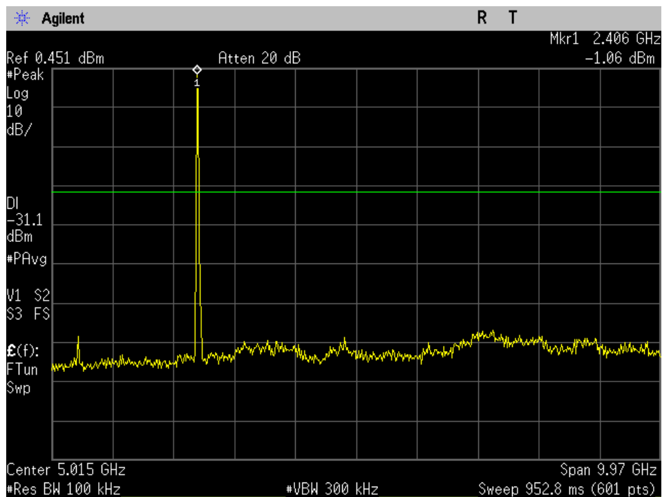
WIFI_Low Ch_2412MHz_20MHz BW_n-mode_-30dBc_30MHz-10GHz_Port 1
