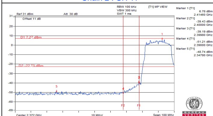
Chain 2 : CH 1 Band edge
