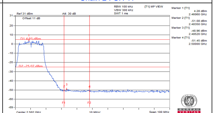
Chain 2 : CH 11 Band edge
