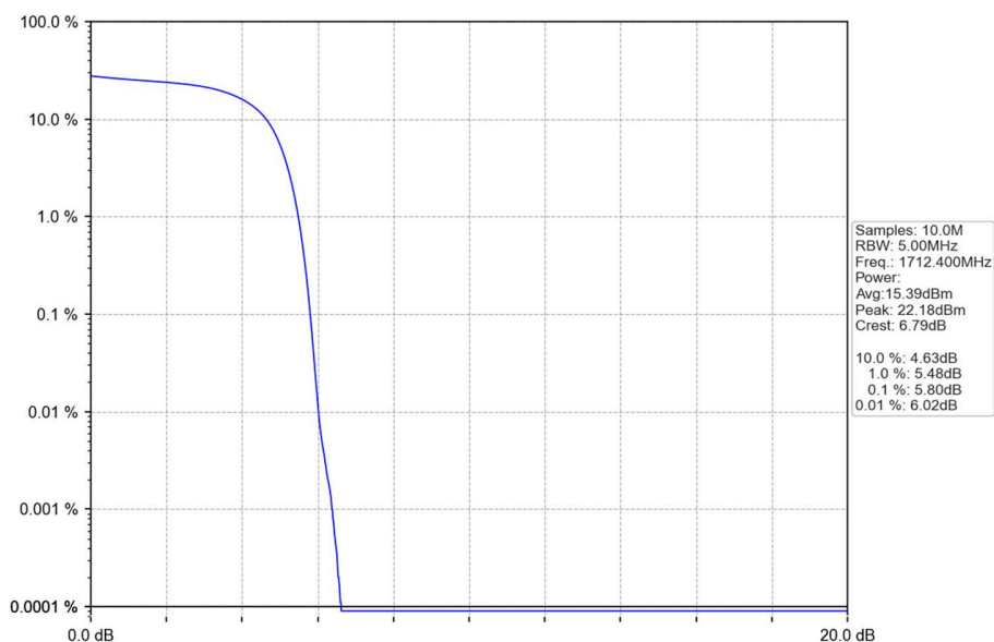
Band4_HSUPA_LCH_1712.4MHz_Subtest 1_NTNV
