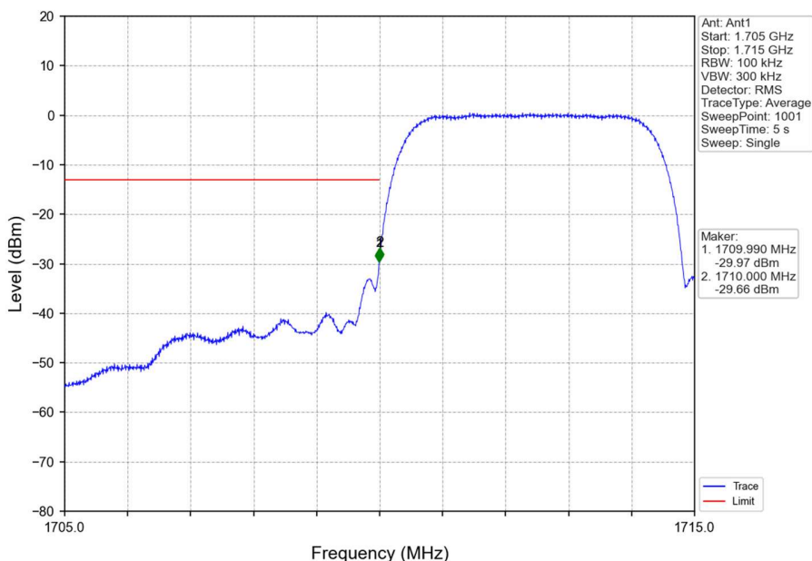
Band4_HSUPA_LCH_1712.4MHz_Subtest 1_NTNV
