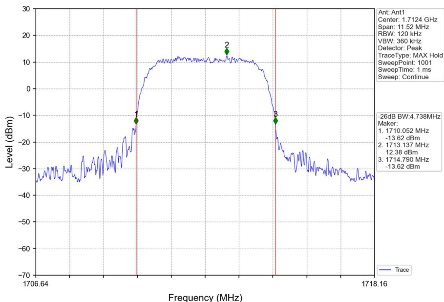
Band4_HSUPA_LCH_1712.4MHz_Subtest 1_NTNV
