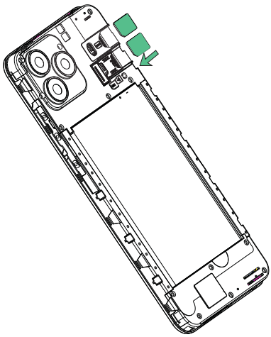
EN Insert SIM card(s) 2
