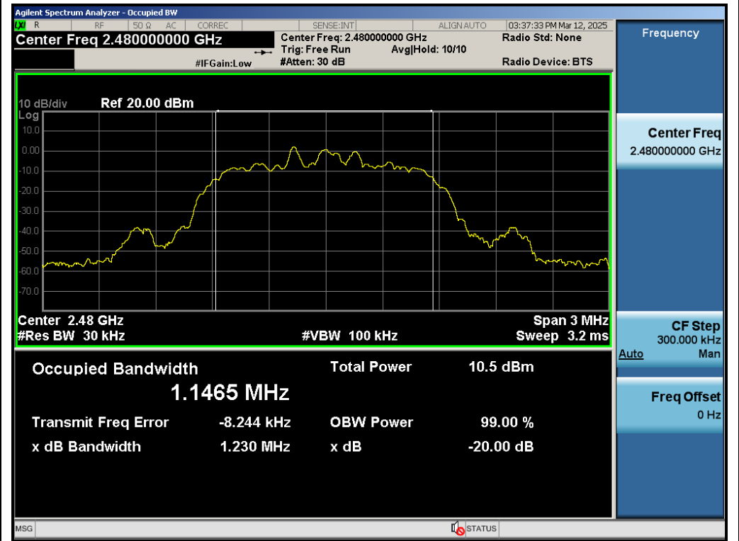
Test_Graph_EDR_ANT1_2480_2Mbps_OBW
