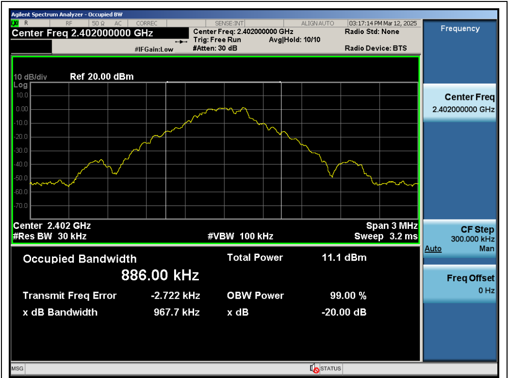
Test_Graph_BR_ANT1_2402_1Mbps_OBW
