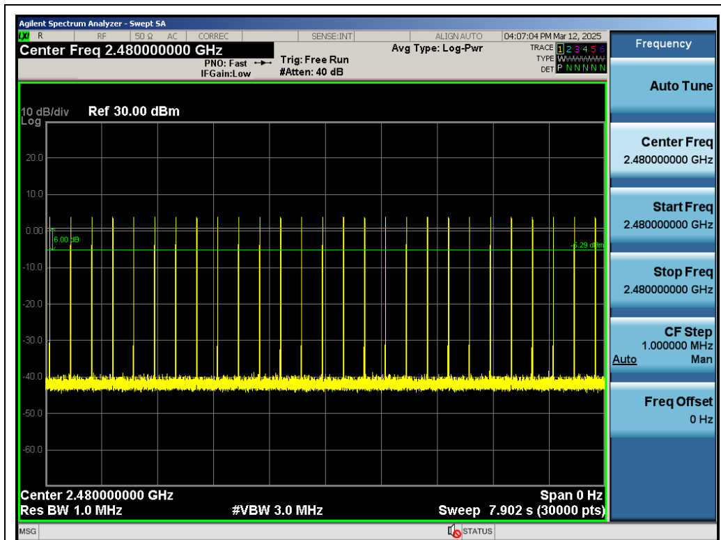
Test_Graph_EDR_HOP_ANT1_NA_3Mbps_2480_Number of Burst
