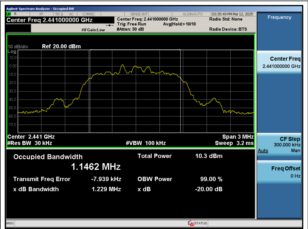
Test_Graph_EDR_ANT1_2441_2Mbps_OBW
