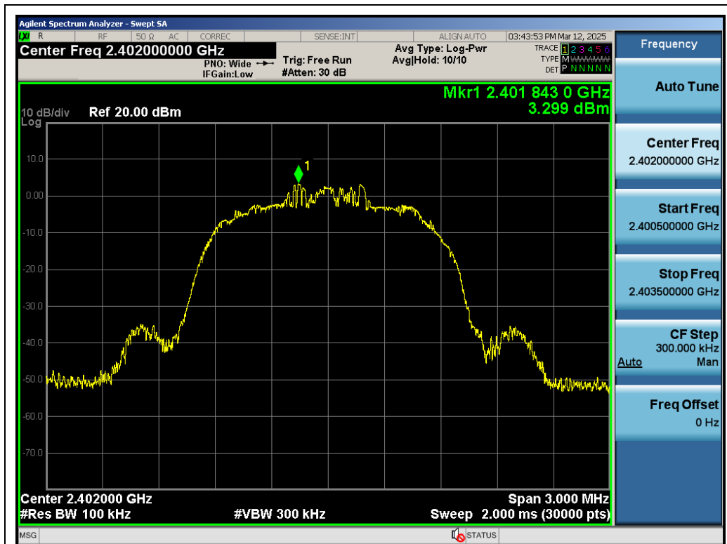
Test_Graph_EDR_ANT1_2402_3Mbps_Reference Level
