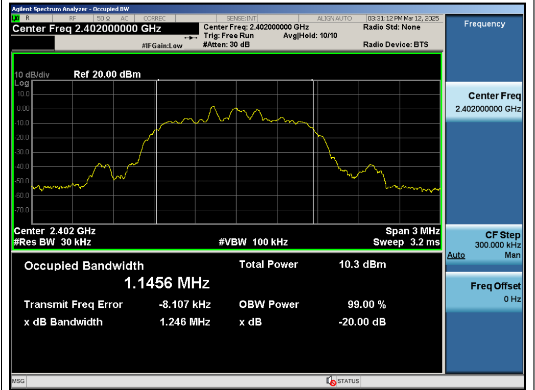
Test_Graph_EDR_ANT1_2402_2Mbps_OBW
