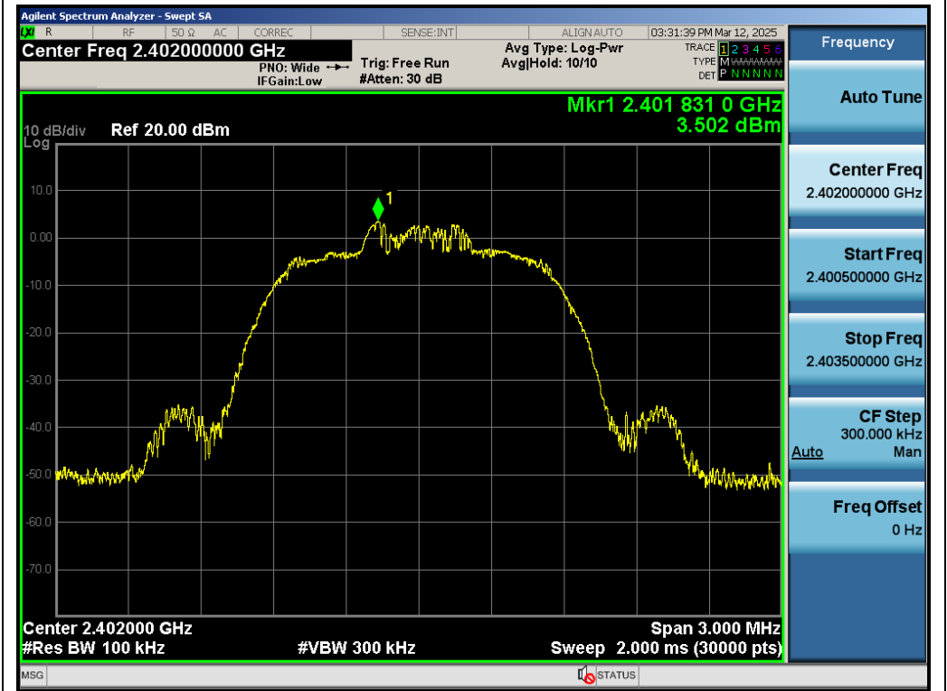
Test_Graph_EDR_ANT1_2402_2Mbps_Reference Level
