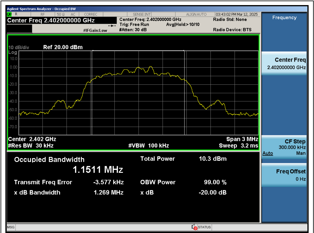
Test_Graph_EDR_ANT1_2402_3Mbps_OBW
