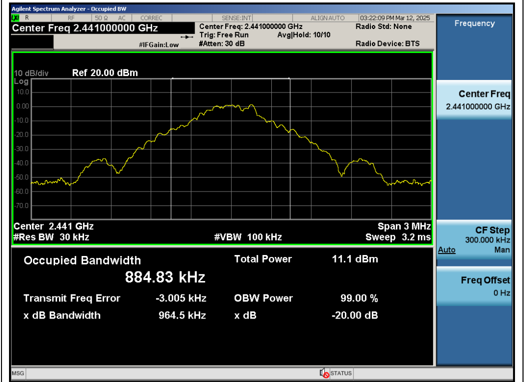
Test_Graph_BR_ANT1_2441_1Mbps_OBW
