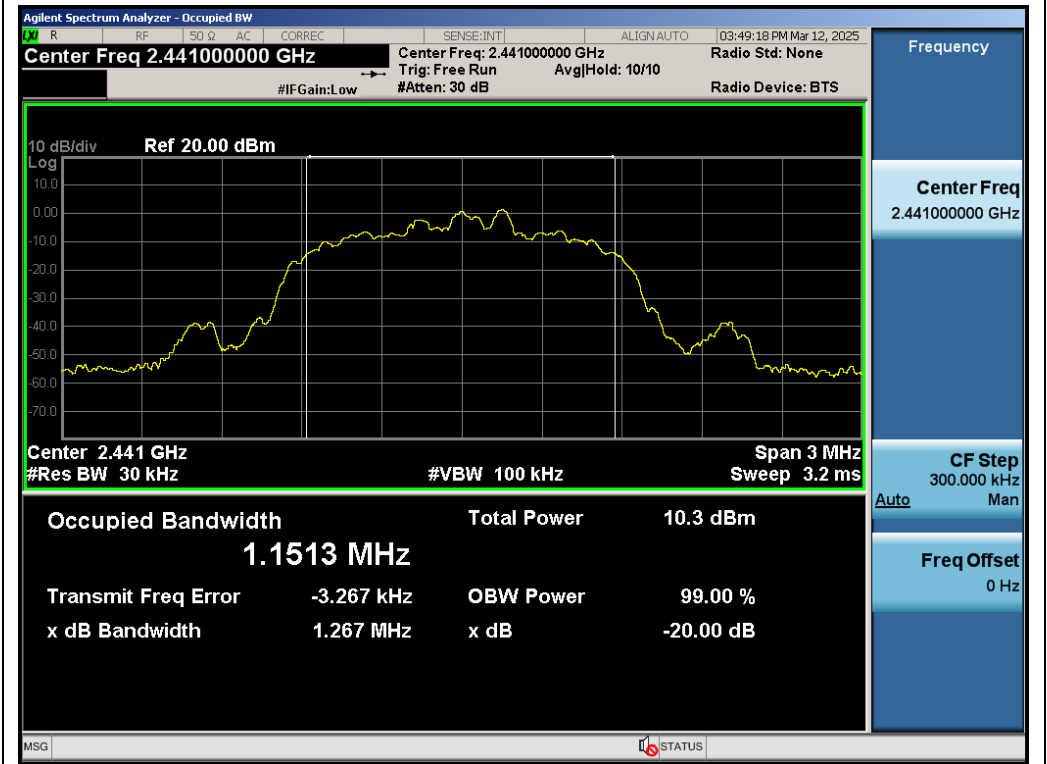
Test_Graph_EDR_ANT1_2441_3Mbps_OBW
