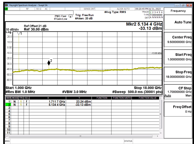
CSE B66 3M CH131987 QPSK(1,7) 1G-18G
