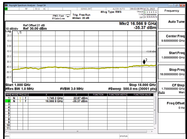
CSE B66 20M CH132322 QPSK(1,50) 1G-18G
