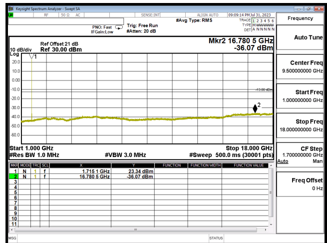
CSE B66 10M CH132022 QPSK(1,25) 1G-18G
