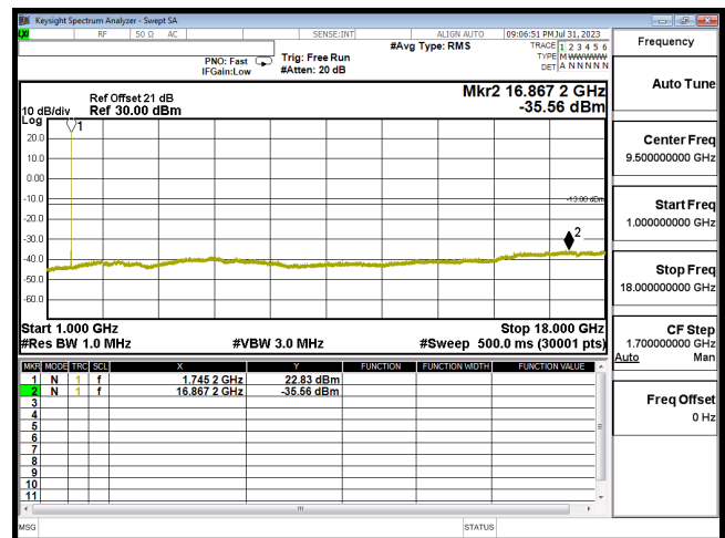
CSE B66 15M CH132322 QPSK(1,37) 1G-18G
