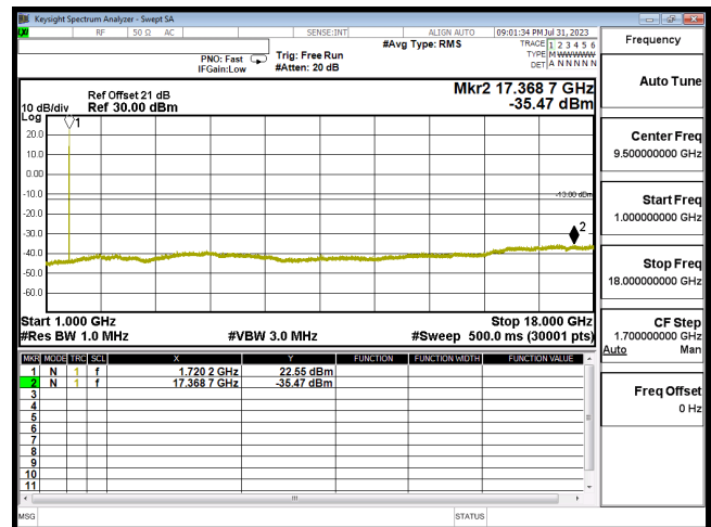
CSE B66 20M CH132072 QPSK(1,50) 1G-18G
