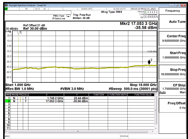
CSE B66 3M CH132322 QPSK(1,7) 1G-18G
