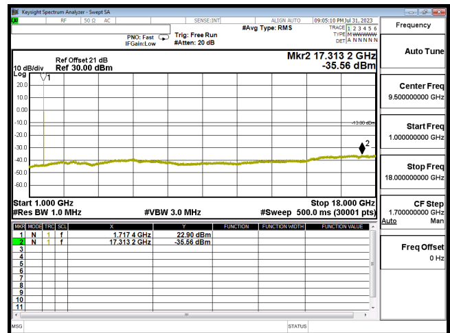
CSE B66 15M CH132047 QPSK(1,37) 1G-18G
