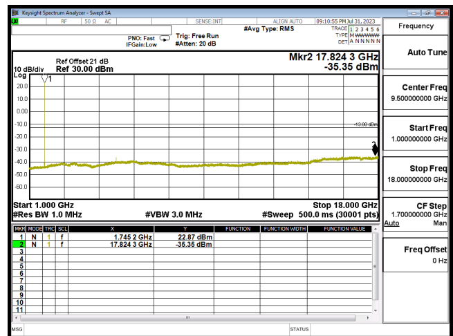
CSE B66 10M CH132322 QPSK(1,25) 1G-18G
