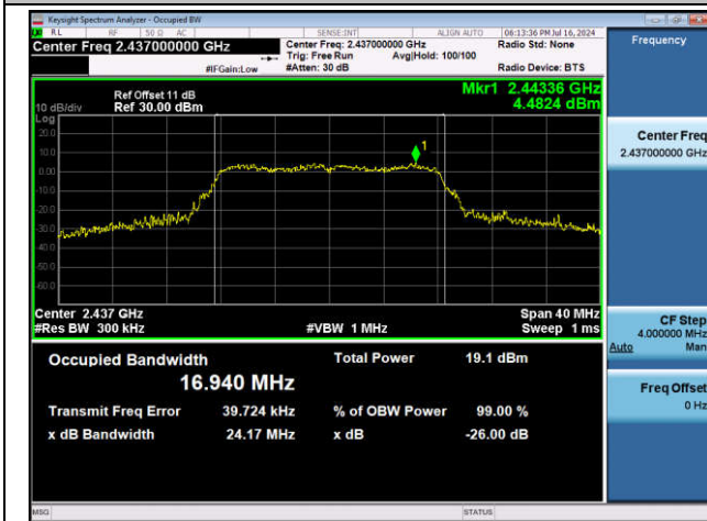
11G-Ant1-2437
