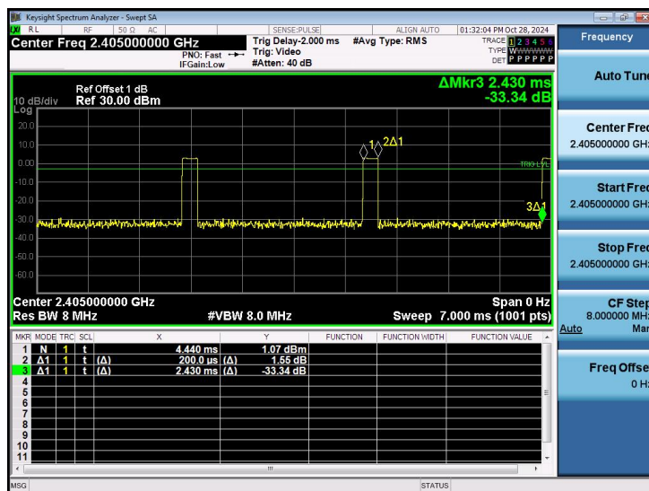
NTNV-2.4G-Ant1-2405
