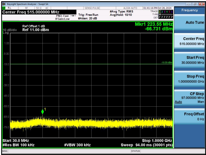
2.4G-Ant1-2475-30~1000-PASS
