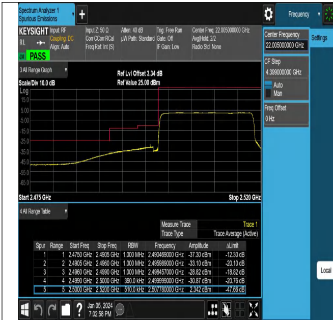
NTNV_N7_PC3_15_20_L_TID1_#1
