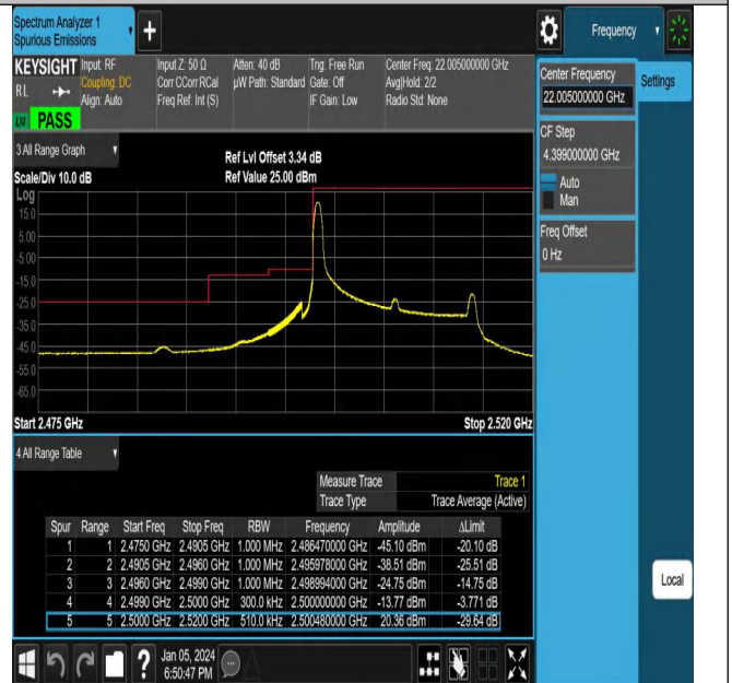
NTNV_N7_PC3_15_15_L_TID11_#1
