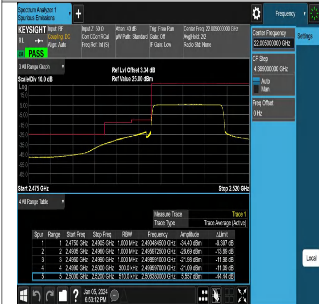
NTNV_N7_PC3_15_15_L_TID16_#1
