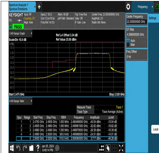
NTNV_N7_PC3_15_15_L_TID1_#1
