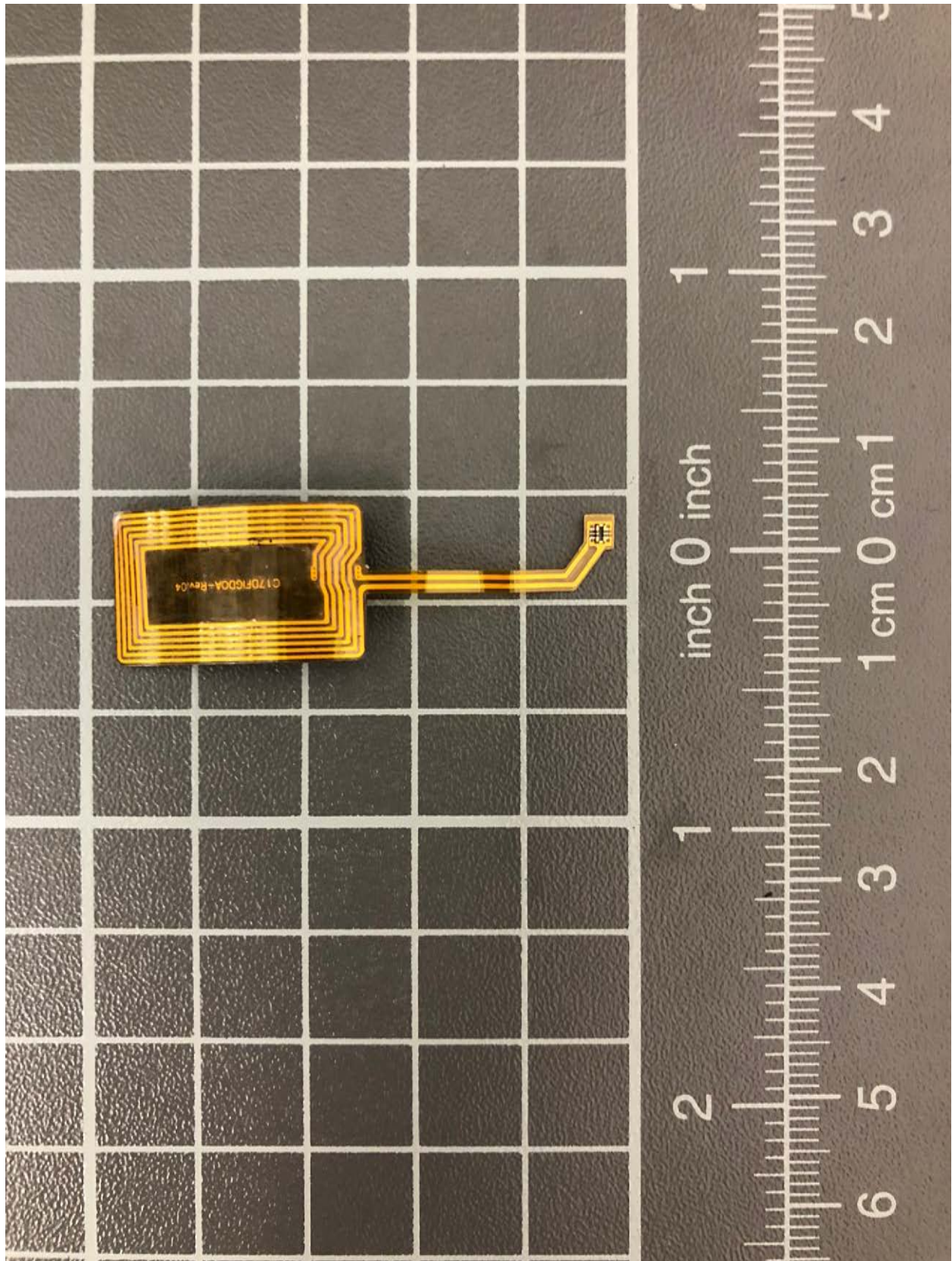
NFC Loop antenna
