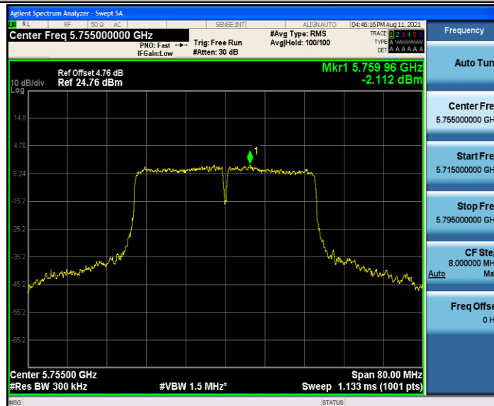
11N40MIMO_Ant2_5755
