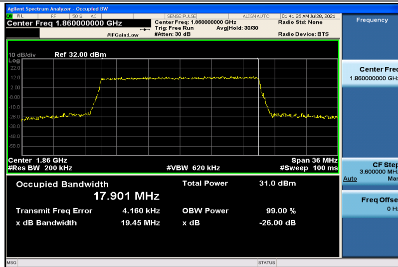
Band2-20MHz-QPSK-18700-100RB#0-17.901
