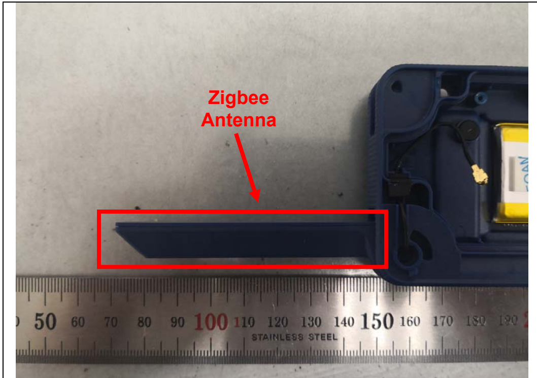
Antenna
