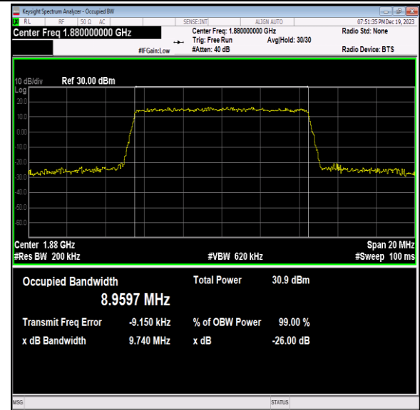
Band2-10MHz-16QAM-18900-50RB#0-PASS
