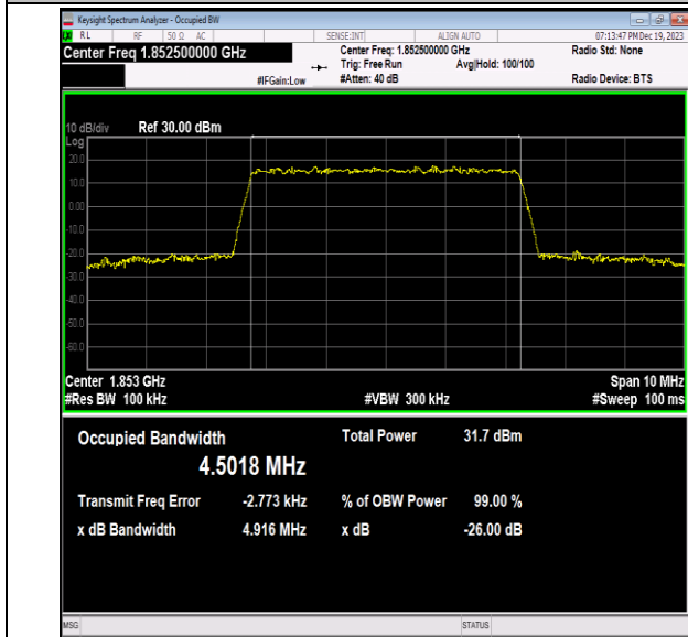
Band2-5MHz-QPSK-18625-25RB#0-PASS
