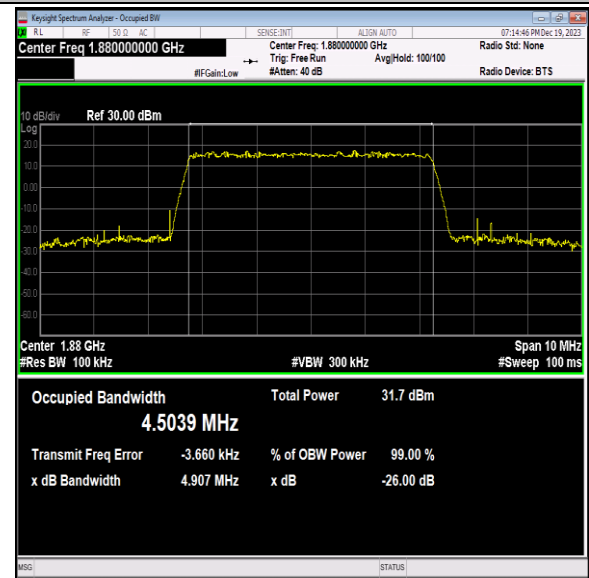
Band2-5MHz-QPSK-18900-25RB#0-PASS
