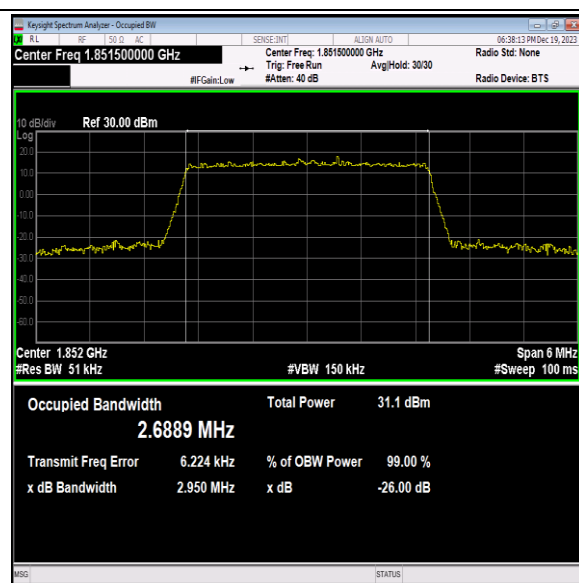
Band2-3MHz-QPSK-18615-15RB#0-PASS
