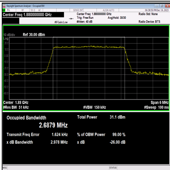
Band2-3MHz-QPSK-18900-15RB#0-PASS
