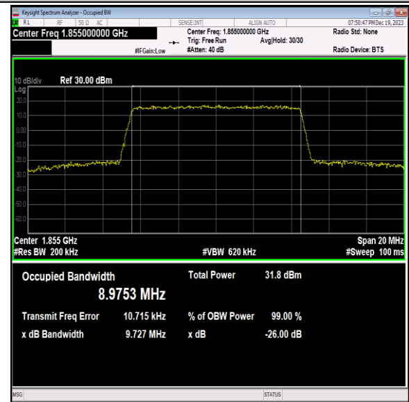
Band2-10MHz-QPSK-18650-50RB#0-PASS
