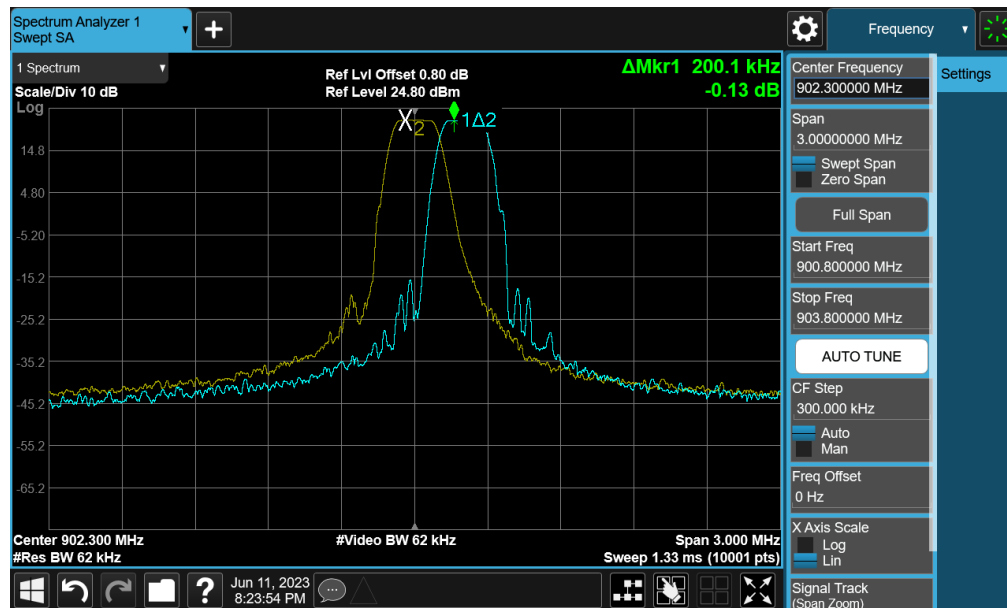
Channel0 902.3MHz
