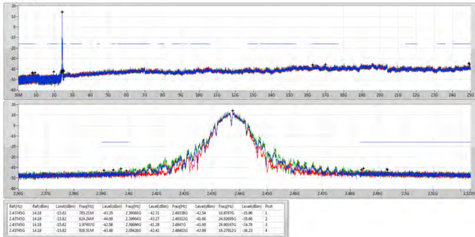
802.11b_Nss1,(1Mbps)_4TX 2437MHz
