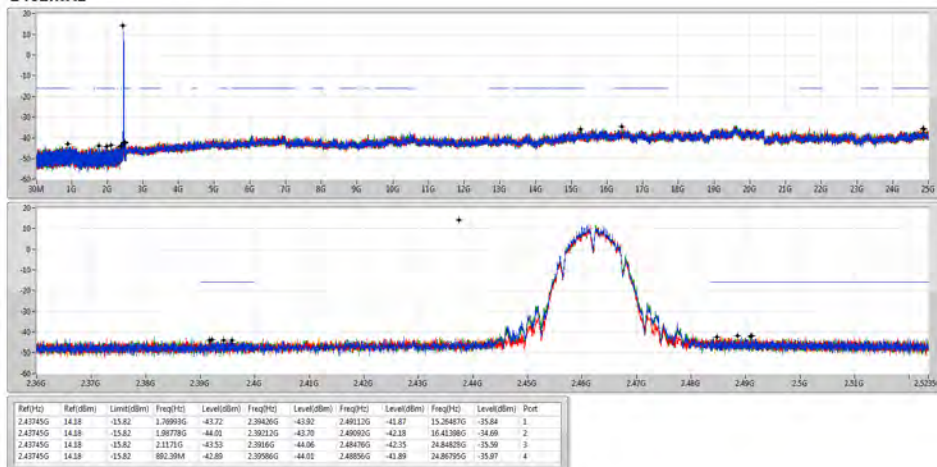
802.11b_Nss1,(1Mbps)_4TX 2462MHz
