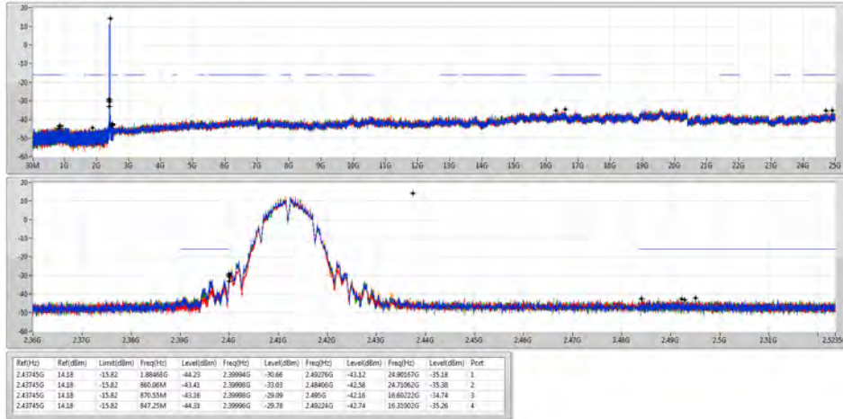
802.11b_Nss1,(1Mbps)_4TX 2412MHz
