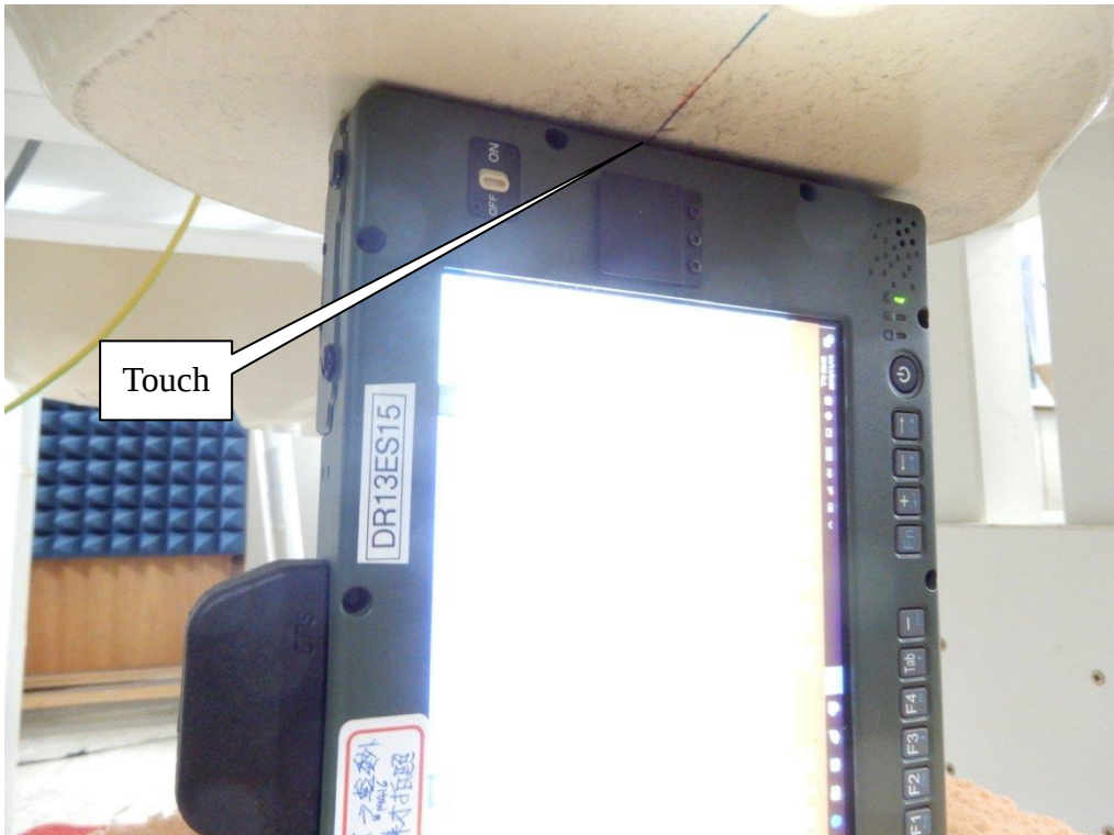
EUT Right-side-Aux
